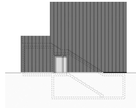
Ansicht Süd
