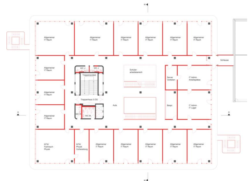
Grundriss 3. Obergeschoss
