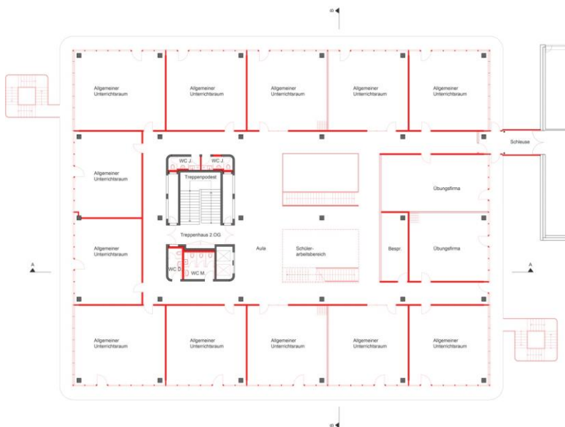
Grundriss 2. Obergeschoss
