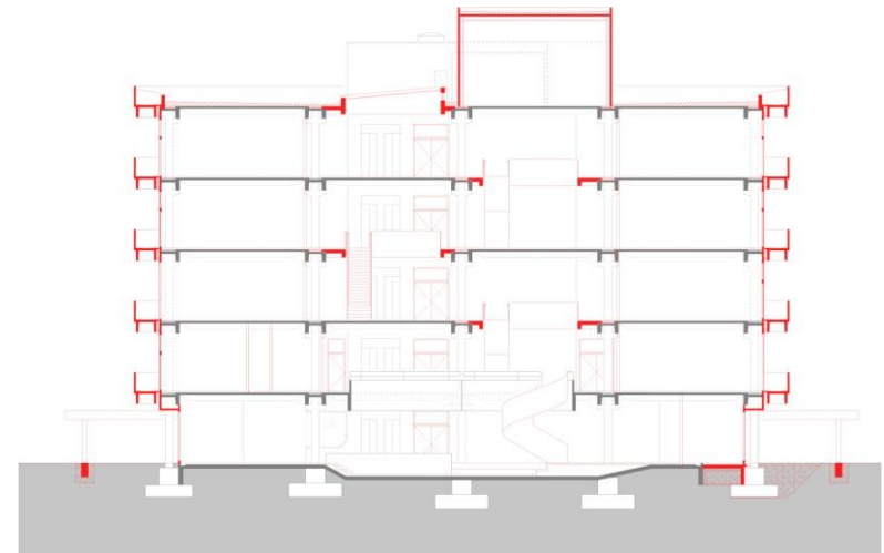
Schnitt B-B
