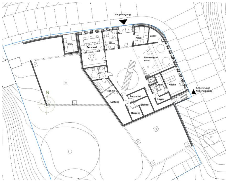
Eingangsebene
