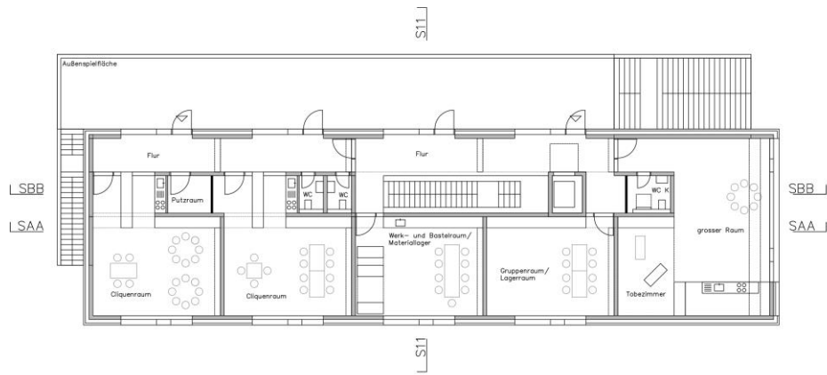
Obergeschoss
