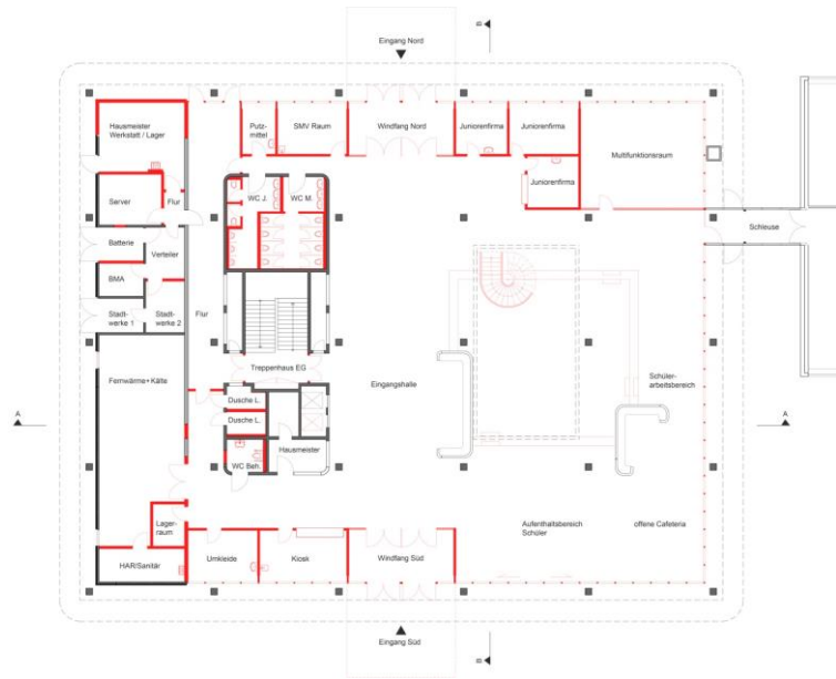
Grundriss Erdgeschoss
