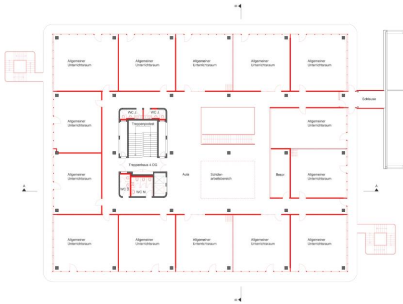
Grundriss 4. Obergeschoss
