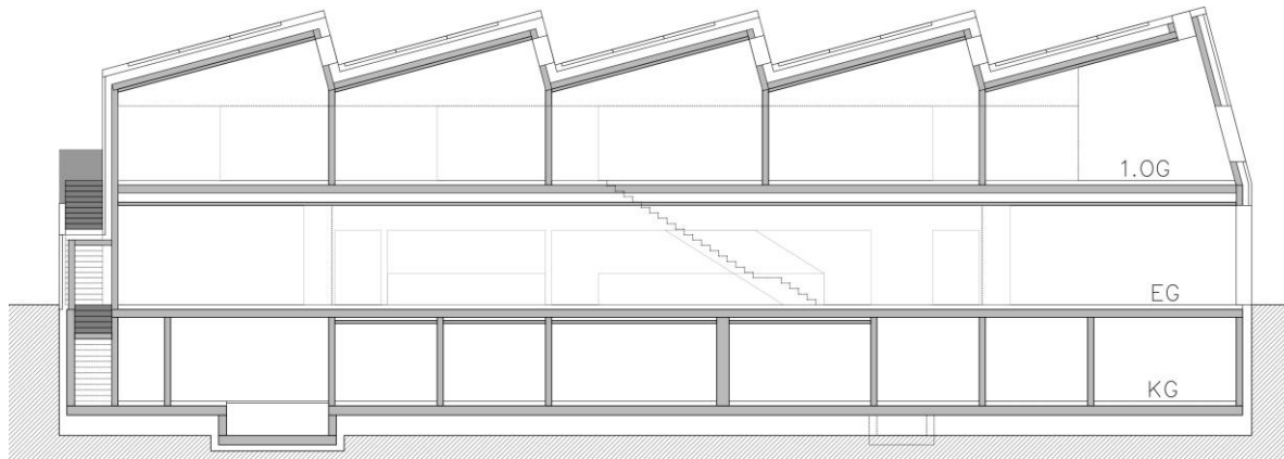
Längsschnitt A-A
