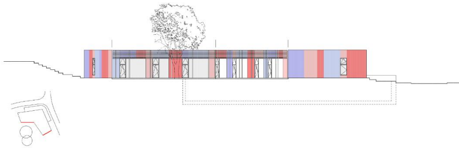
Gartenansicht Süd-Ost
