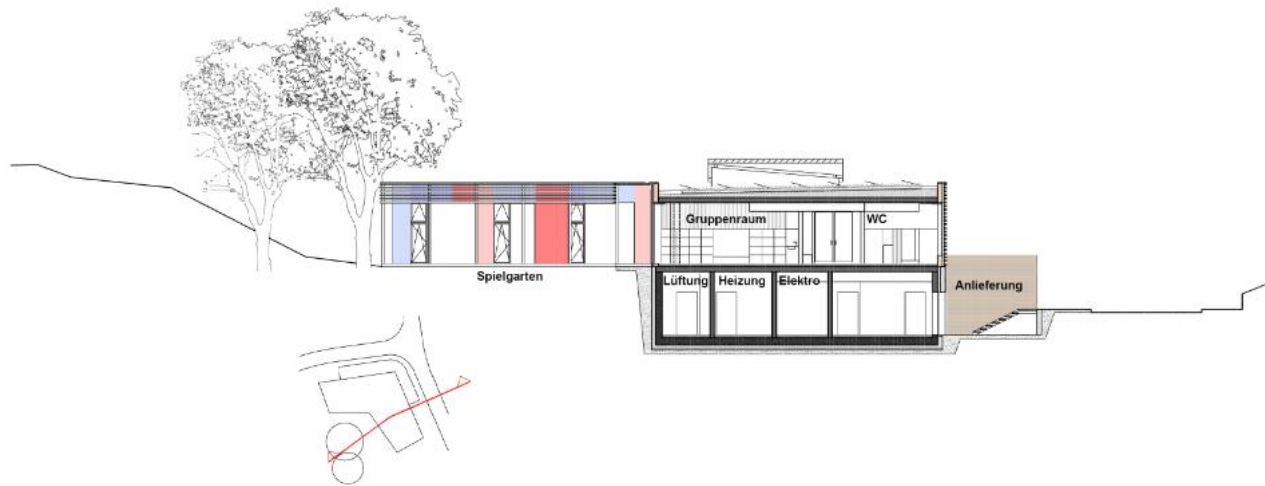
Schnitt B-B
