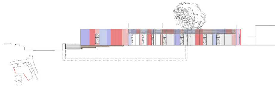
Gartenansicht West
