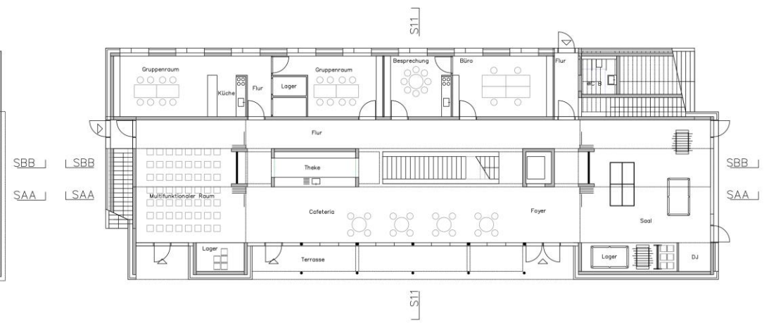
Erdgeschoss
