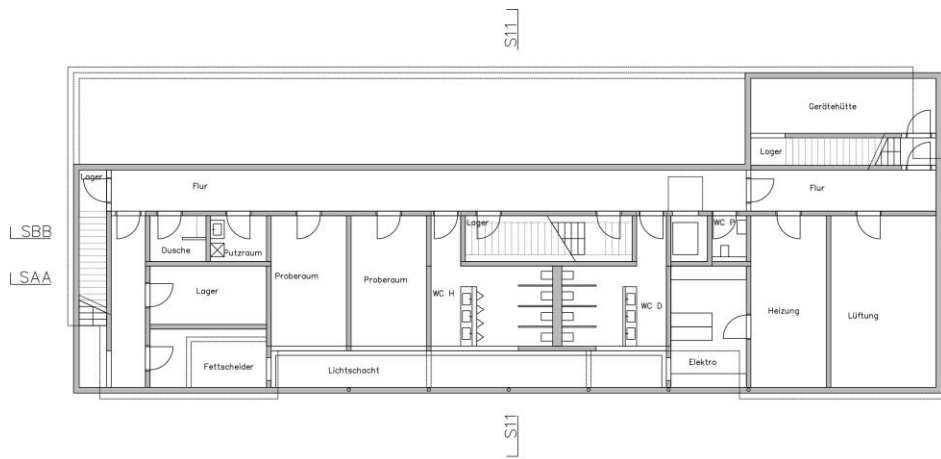
Untergeschoss
