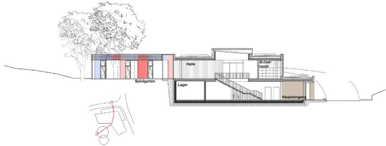
Schnitt A-A
