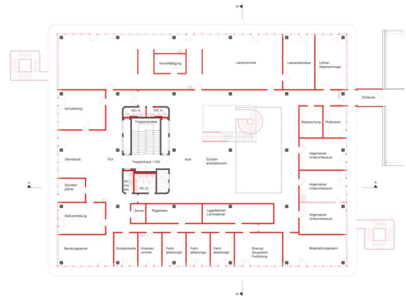
Grundriss 1. Obergeschoss
