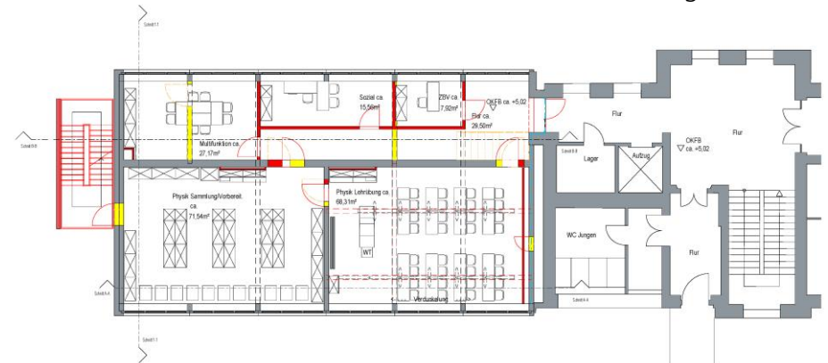
1. Obergeschoss
