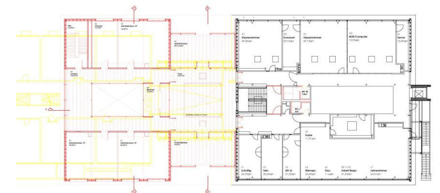
1. Obergeschoss
