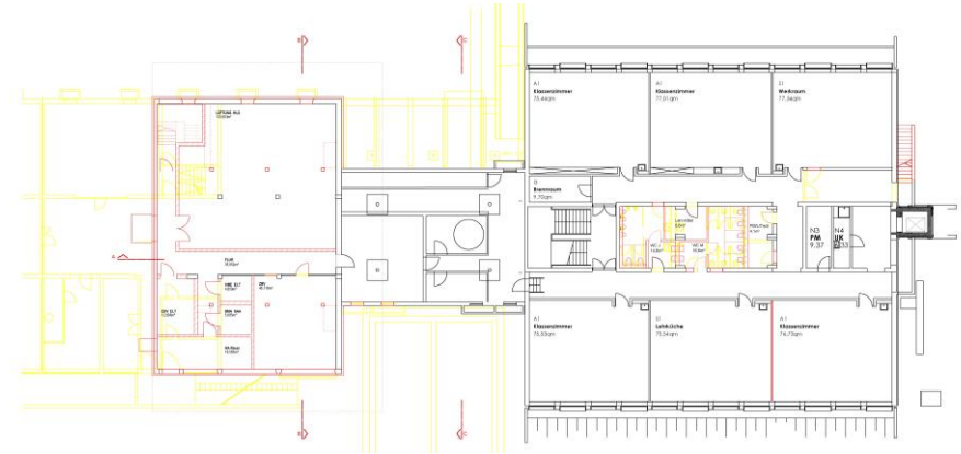
Untergeschoss
