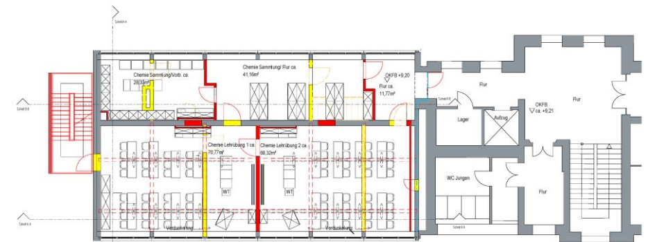
2. Obergeschoss
