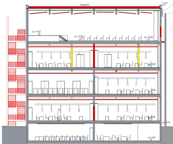
Längsschnitt A-A
