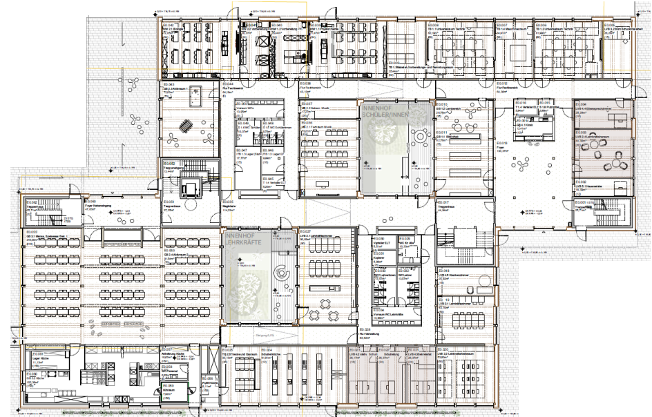
Erdgeschoss
