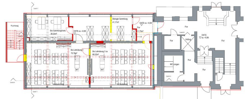
Erdgeschoss
