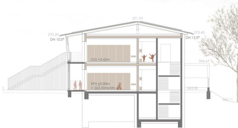
Schnitt B-B
