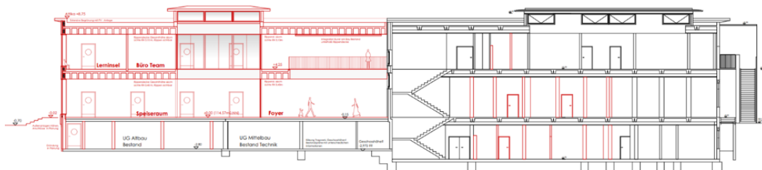
Längsschnitt
