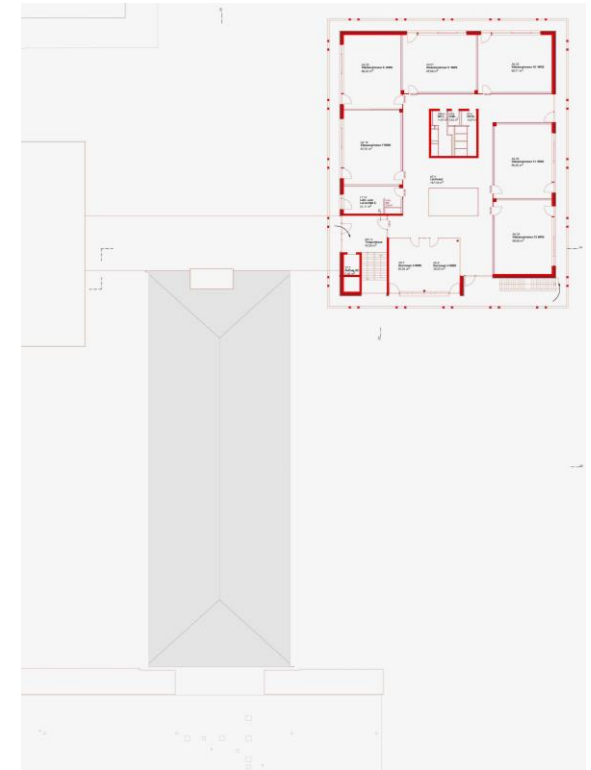
3. Obergeschoss
