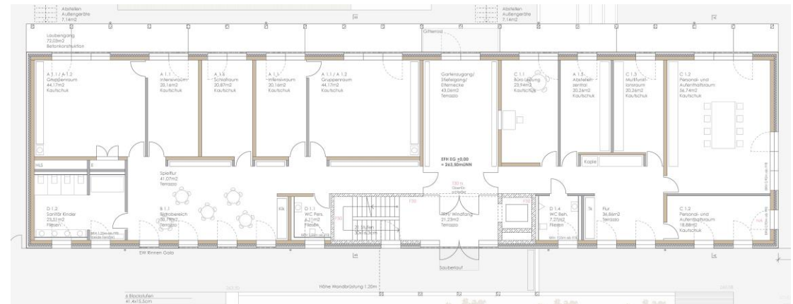
Erdgeschoss
