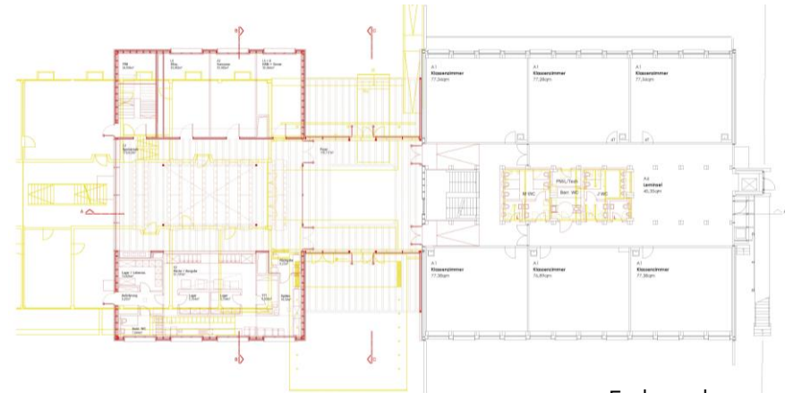
Edgeschoss
