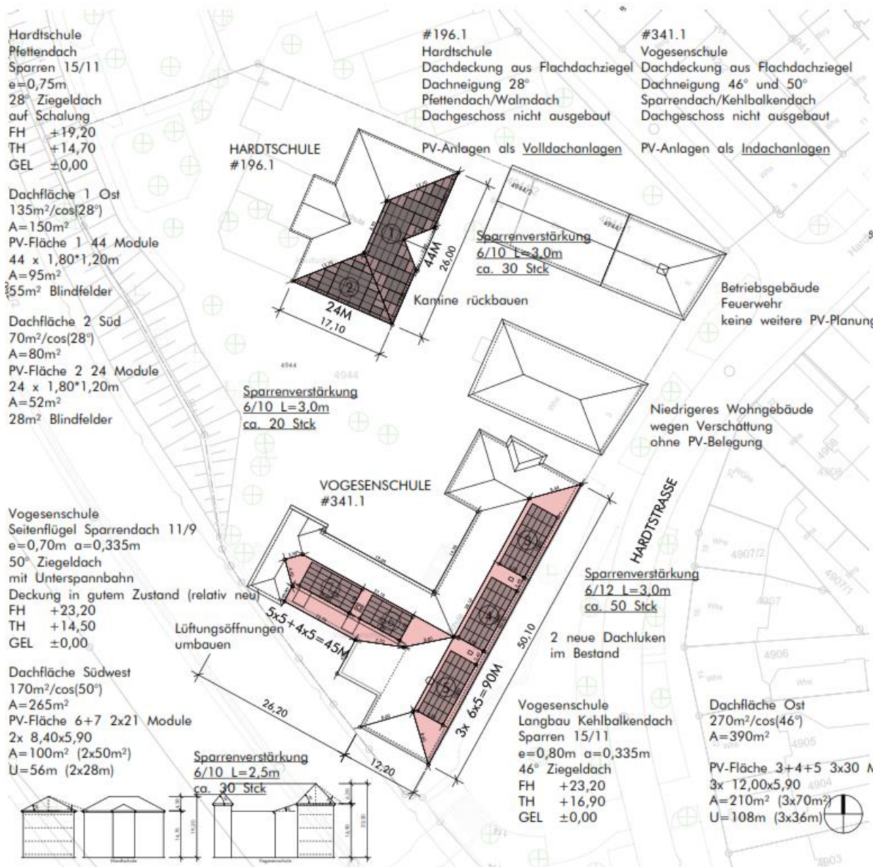
PV-Belegungsplan
