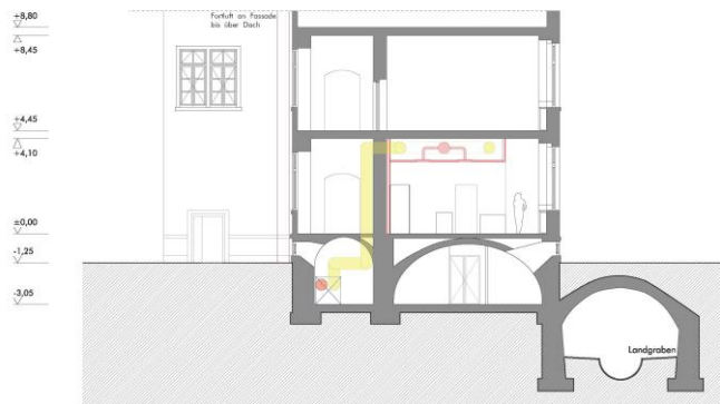
Querschnitt S11
