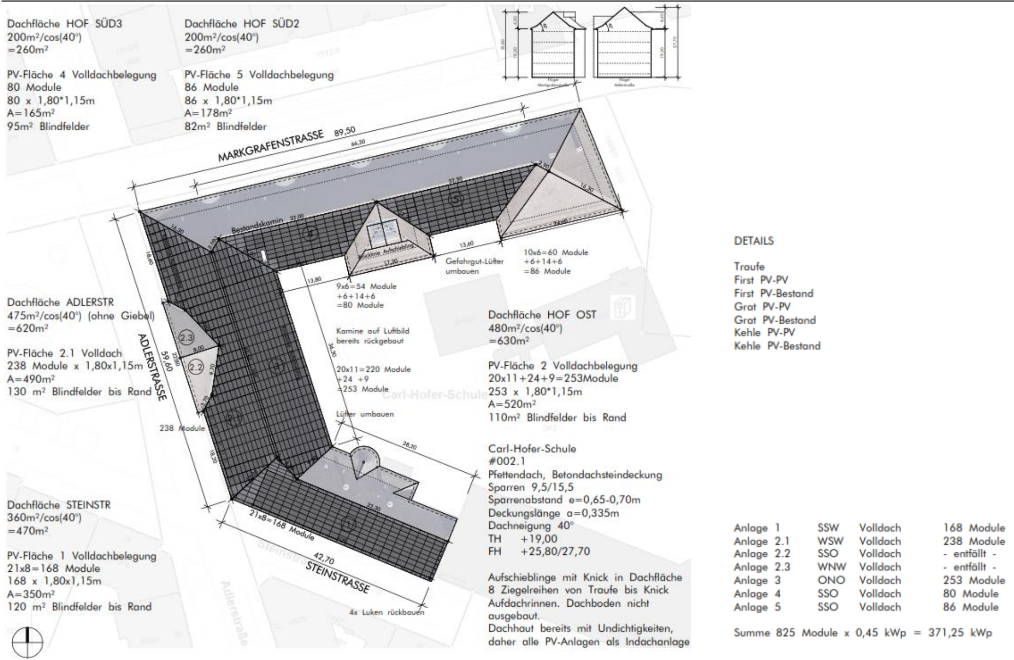
PV-Belegungsplan
