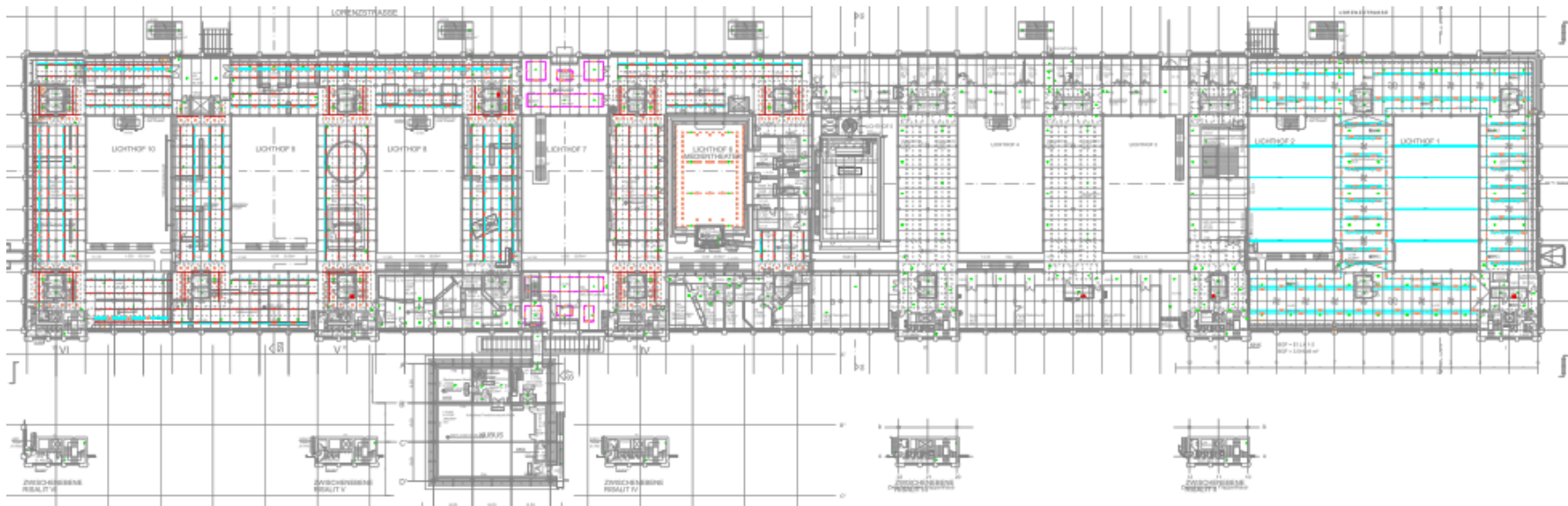
Grundriss 1. Obergeschoss
