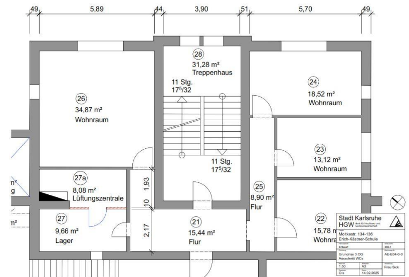
Grundriss 3. OG
