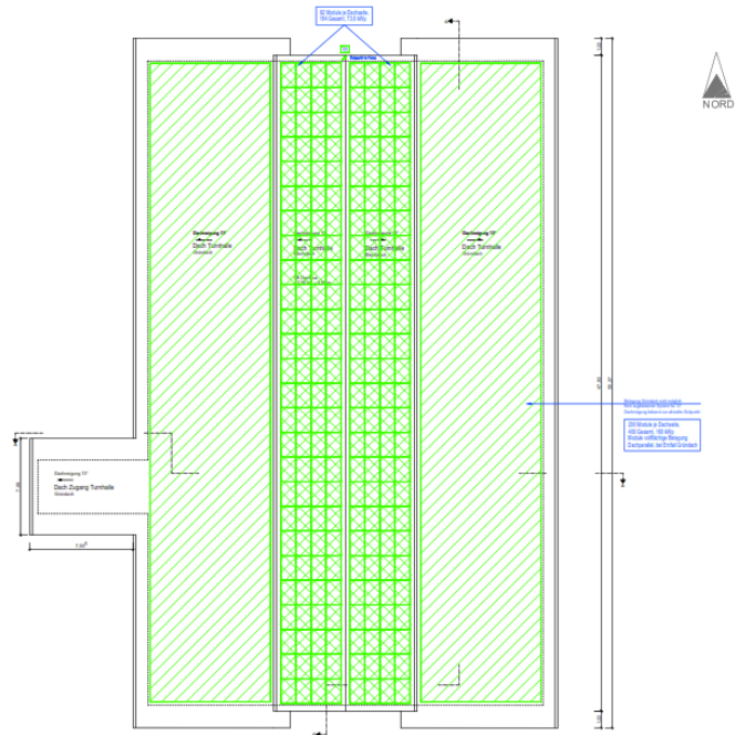
Belegungsplan Turnhalle
