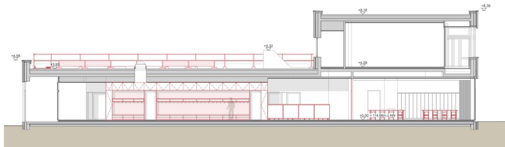
Schnitt C-C
