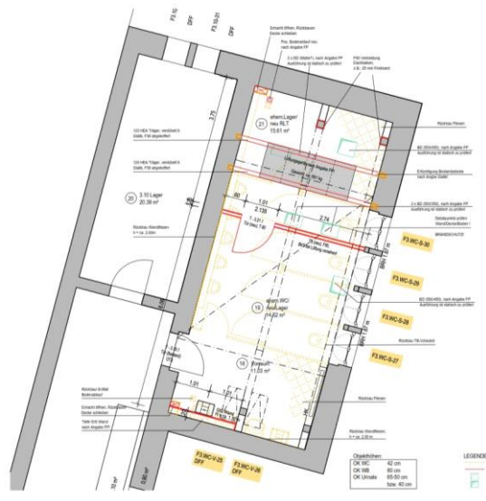
Grundriss Erdgeschoss
