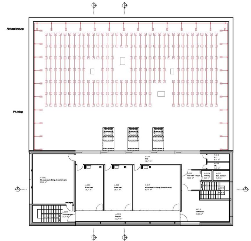
Obergeschoss
