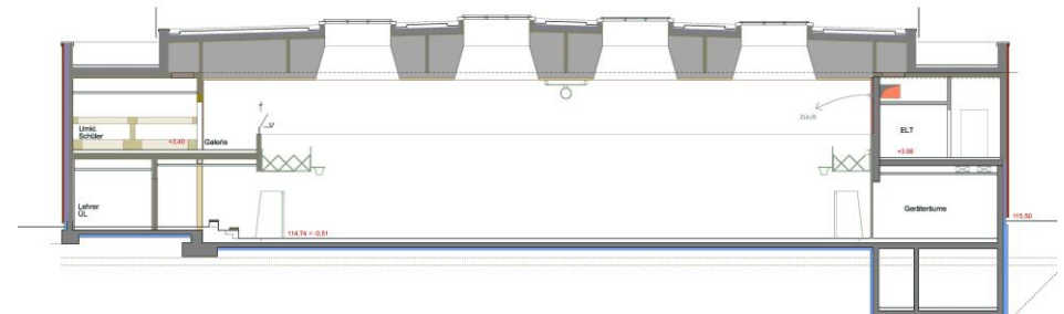
Schnitt 2-2
