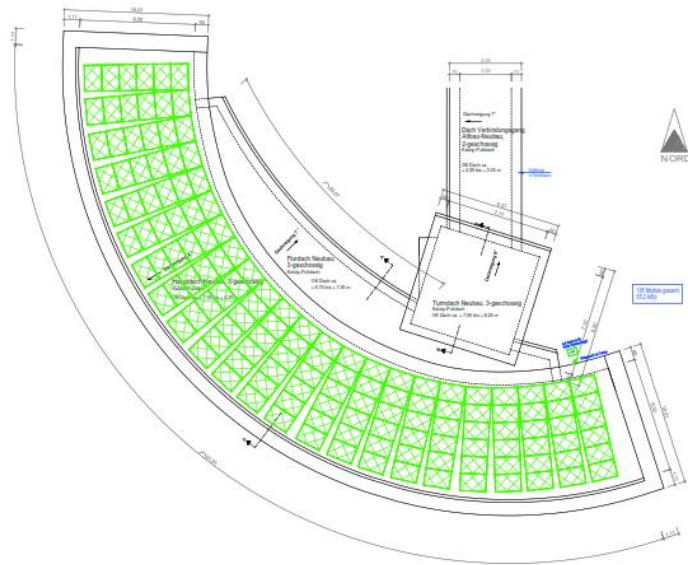
Belegungsplan Neubau
