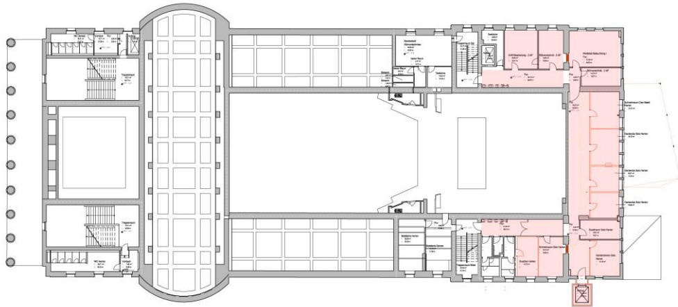
1. Obergeschoss
