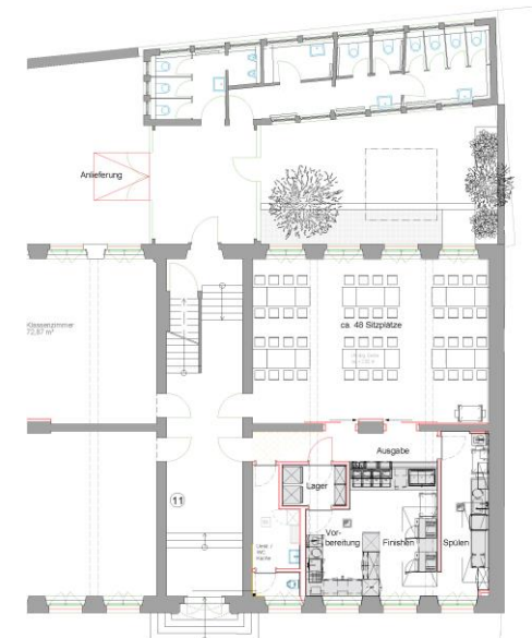
Erdgeschoss - Küchenplanung
