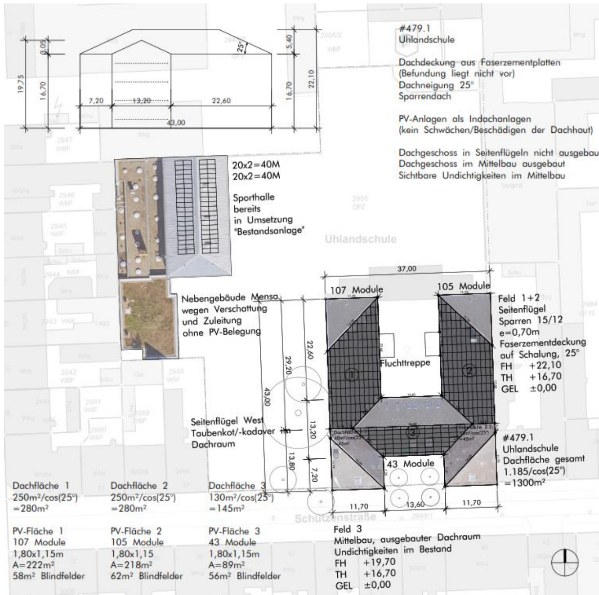
PV-Belegungsplan
