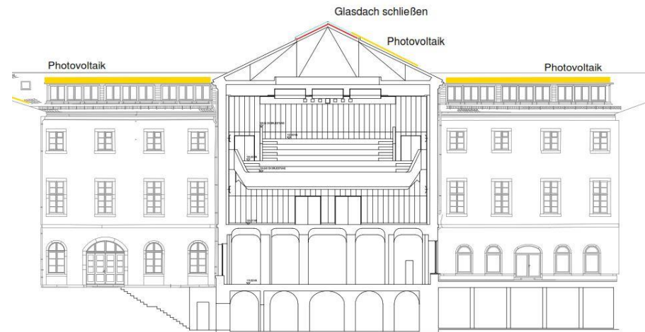
Querschnitt
