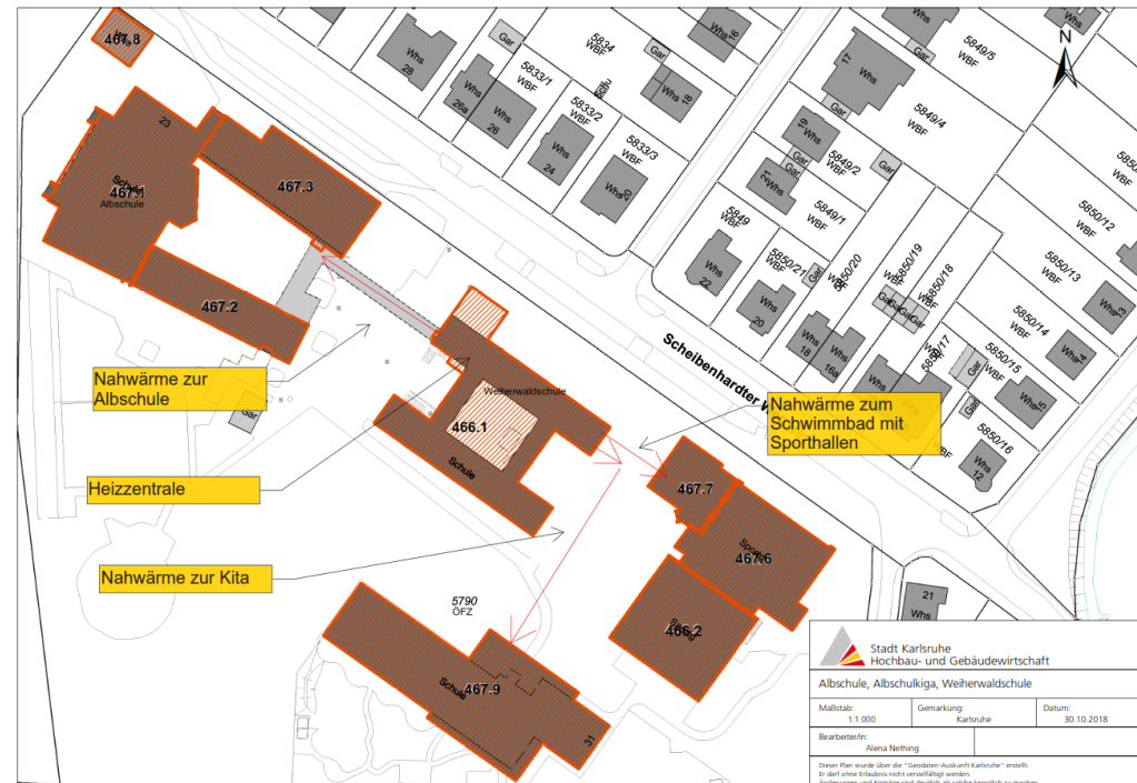
Lageplan Skizze Nahwärmenetz
