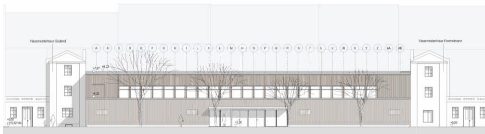
Westansicht
