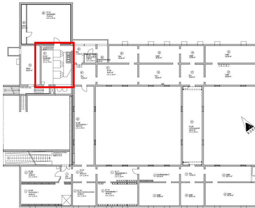
Untergeschoss Heizungsanlage Gaskessel Bestand
