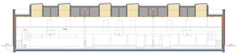
Schnitt 1-1
