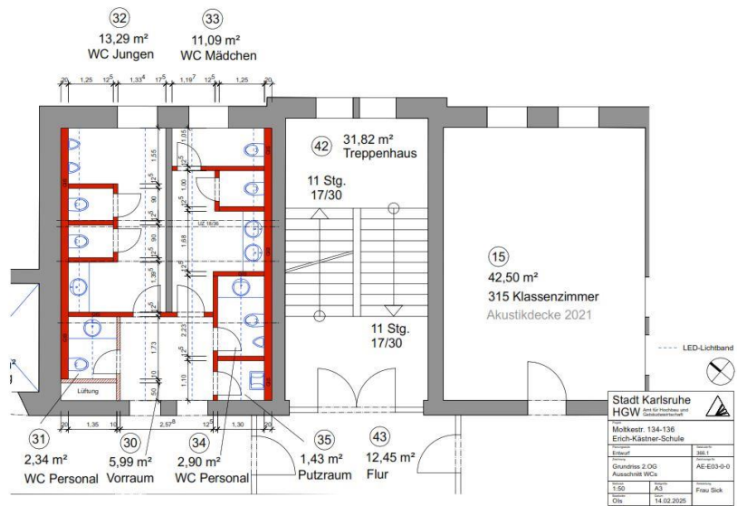
Grundriss 2. OG
