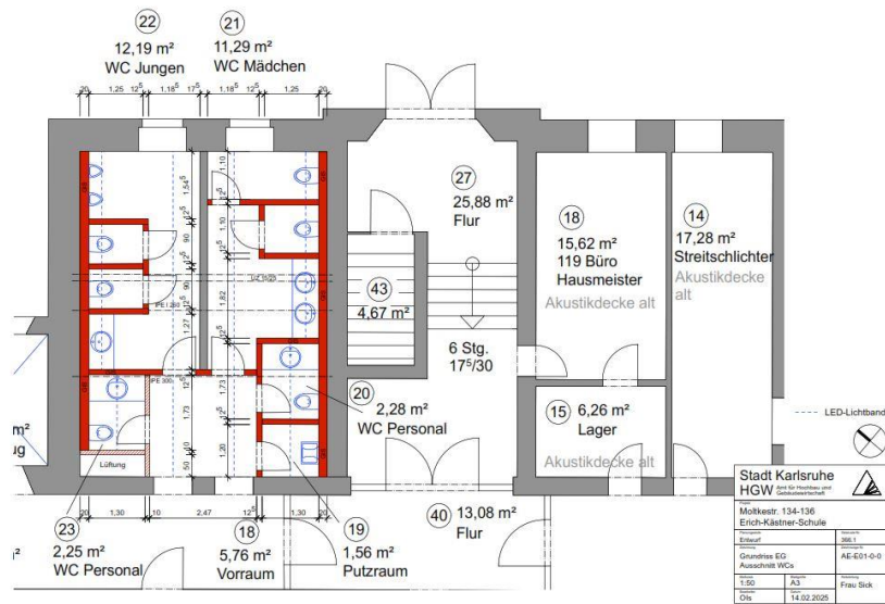
Grundriss EG
