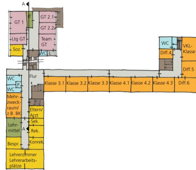
1. Obergeschoss
