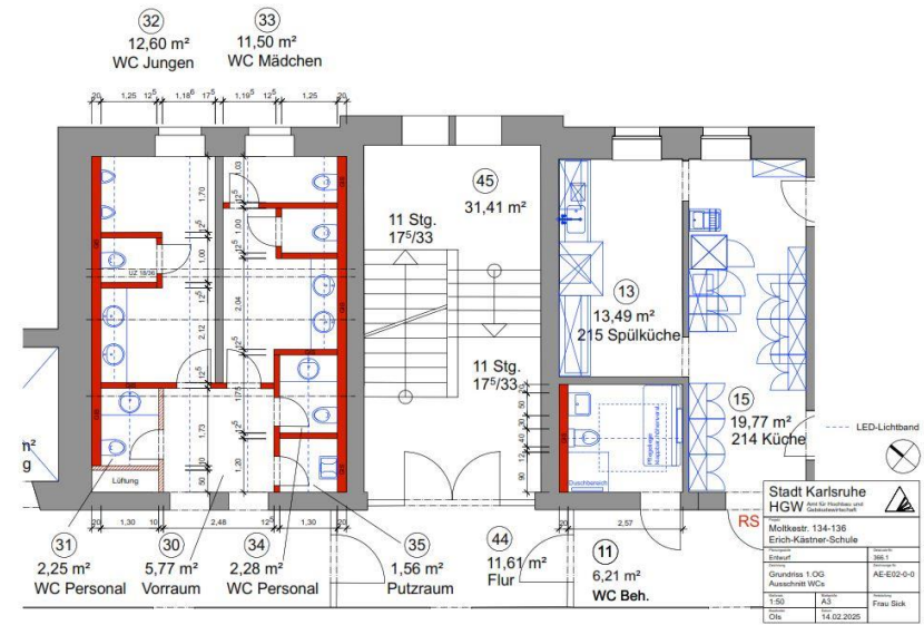
Grundriss 1. OG
