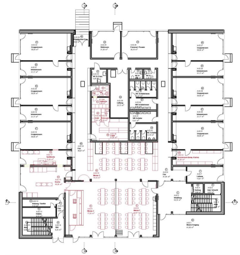
Erdgeschoss
