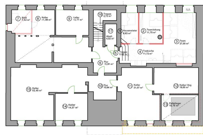
Kellergeschoss
