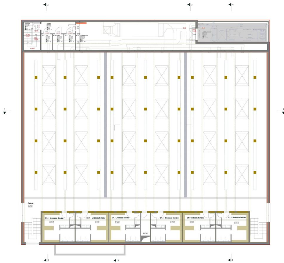
Obergeschoss
