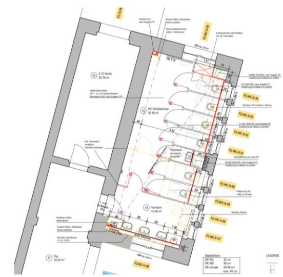
3. Obergeschoss
