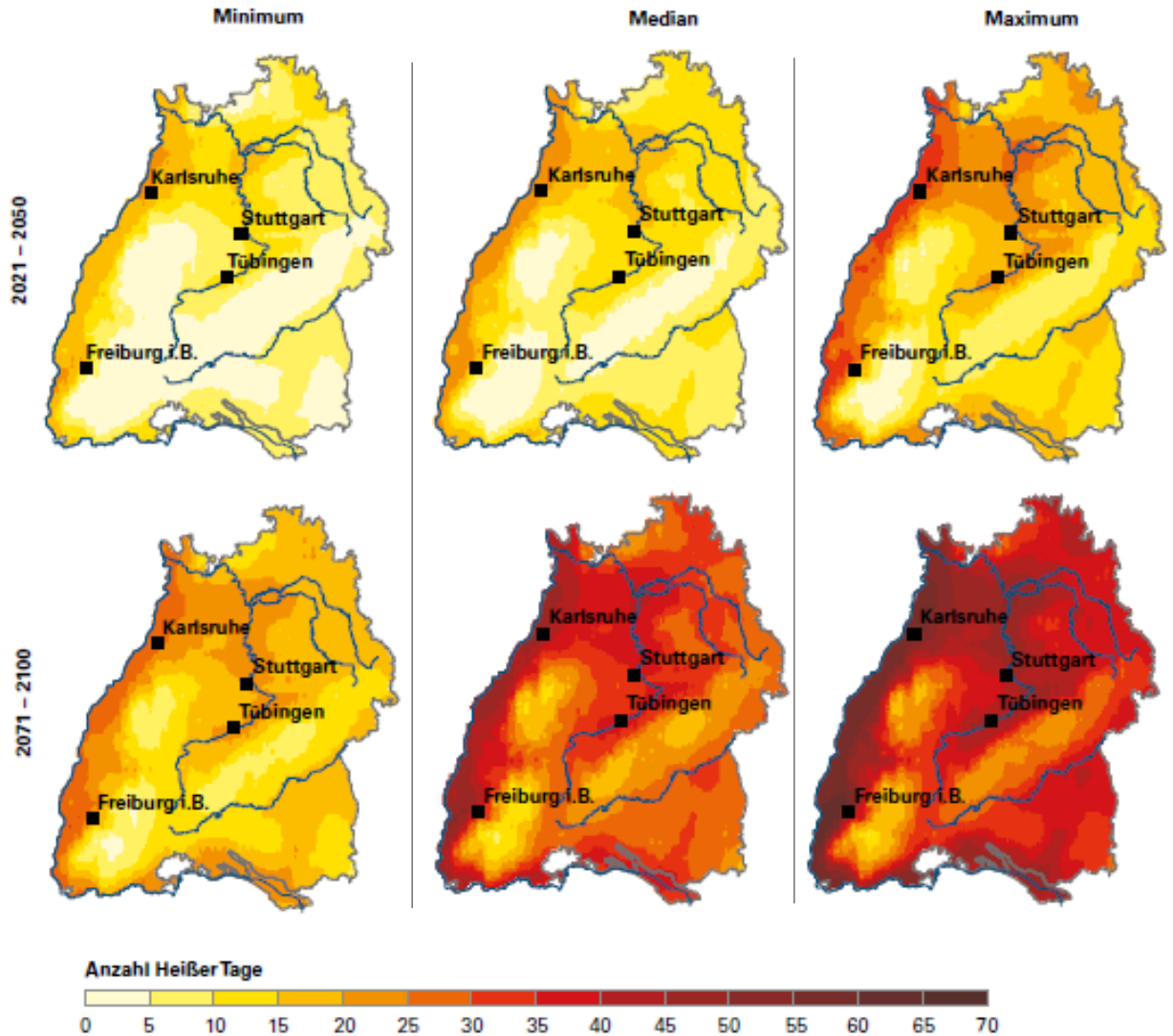
Abbildung 2.6: Anzahl Heißer Tage für die nahe (obere Reihe) und ferne (untere Reihe) Zukunft, Darstellung der Bandbreite für das Ensemble des Szenarios RCP 8.5. Quelle: Modelldaten ReKliEs-De, Auswertung und Darstellung LUBW.
