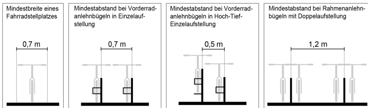
Mindestbreiten/-abstände im Überblick (Schemadarstellung, ohne Maßstab)
