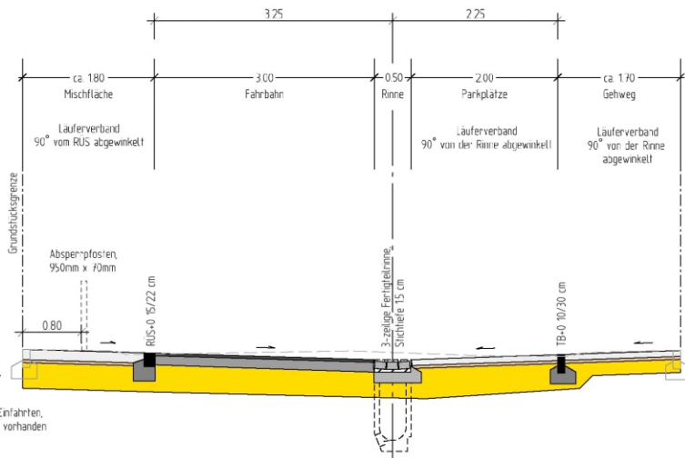
Regelquerschnitt
