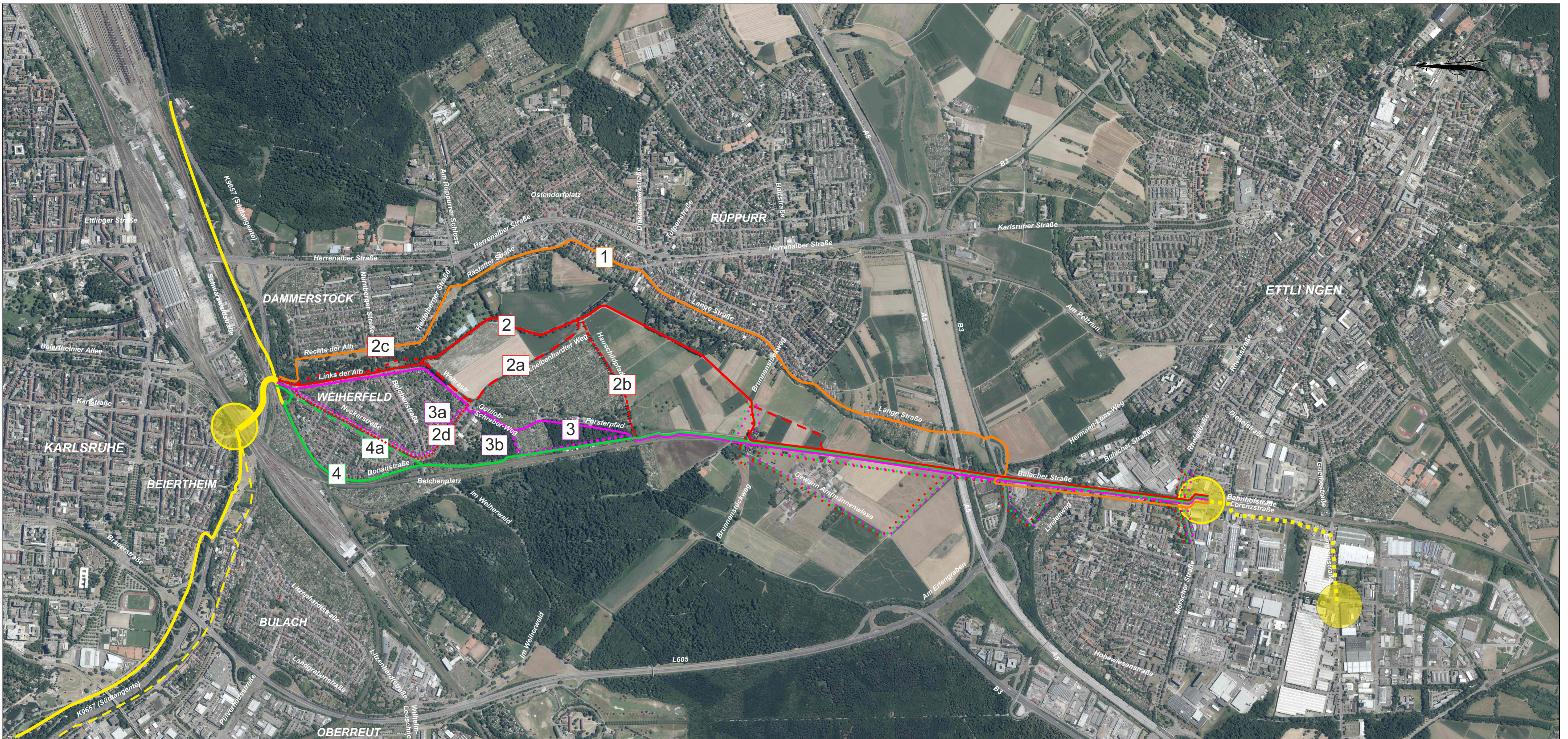
Radschnellverbindung RS 10 Ettlingen-Karlsruhe - Varianten
