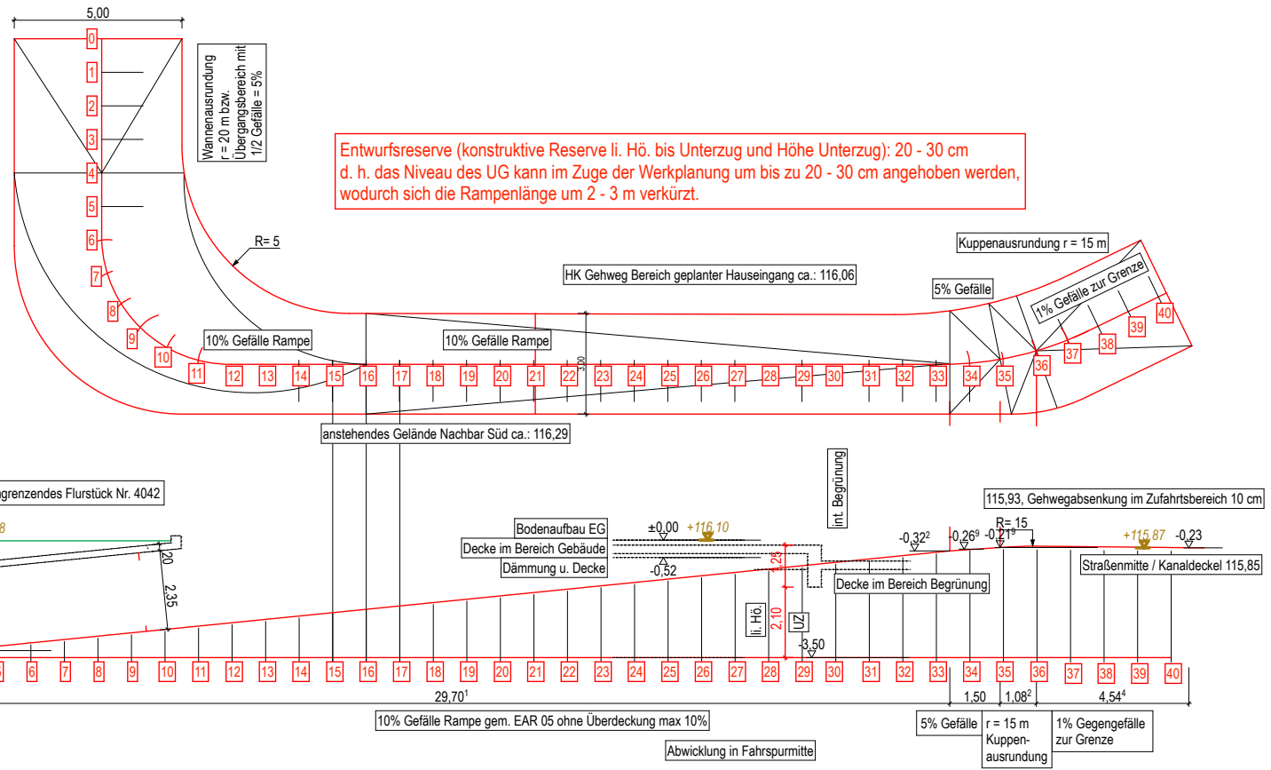
Wichernstr. 4a, Nachweis/Abwicklung Tiefgaragenabfahrt, 2019-03-05
