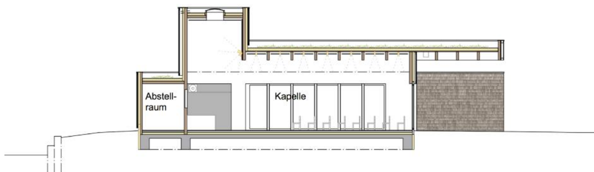
Längsschnitt
