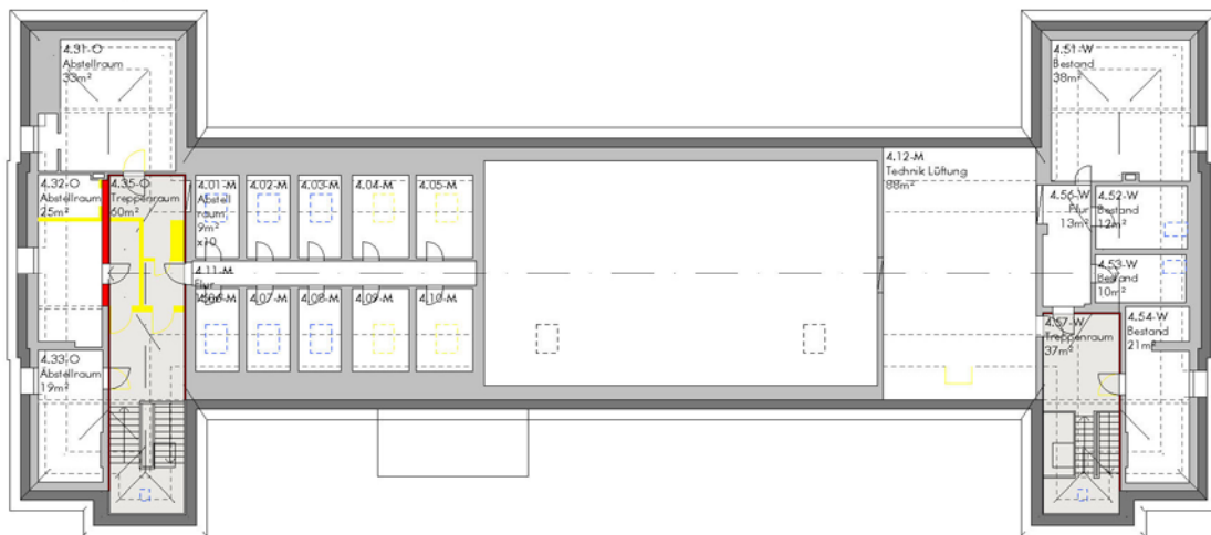
Dachgeschoss
