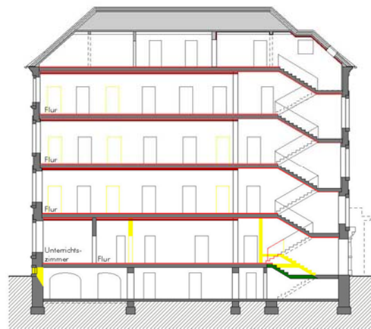
Schnitt D-D
