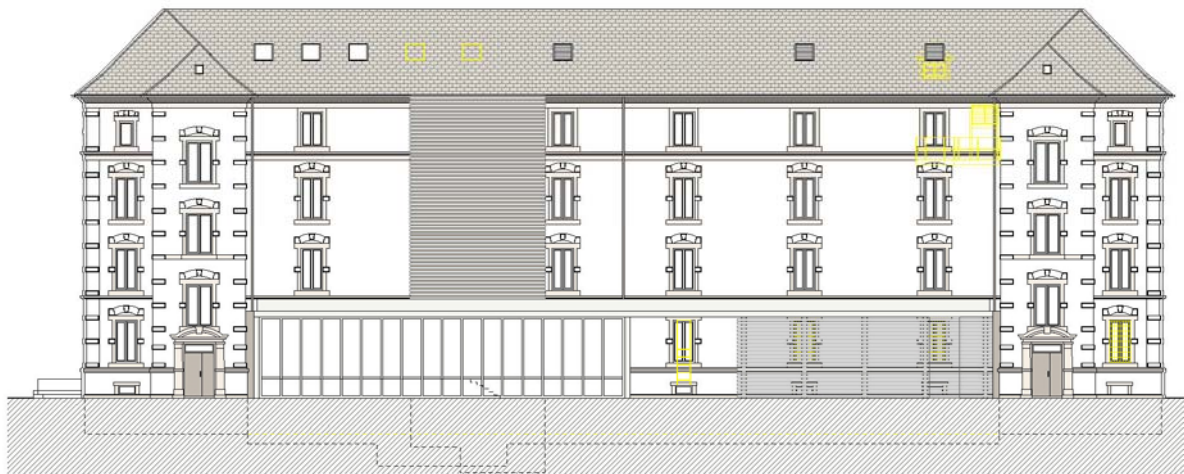
Ansicht Nord
