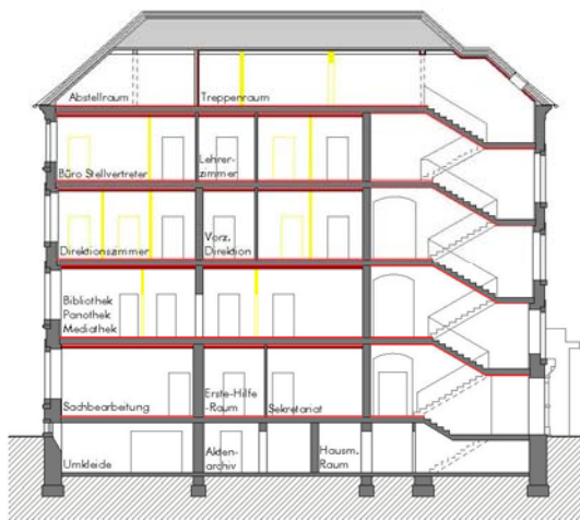
Schnitt A-A
