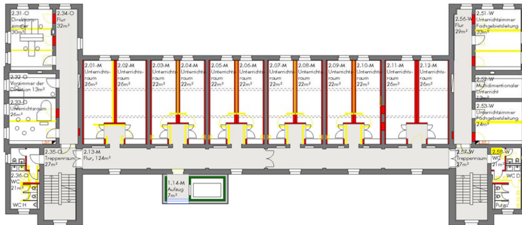
2.Obergeschoss
