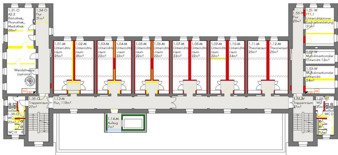
1. Obergeschoss
