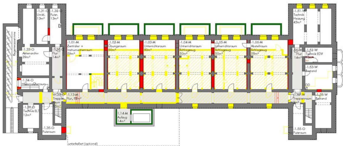
Untergeschoss
