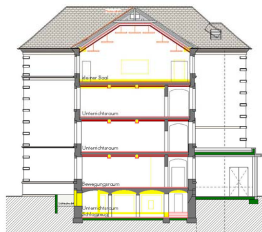
Schnitt C-C
