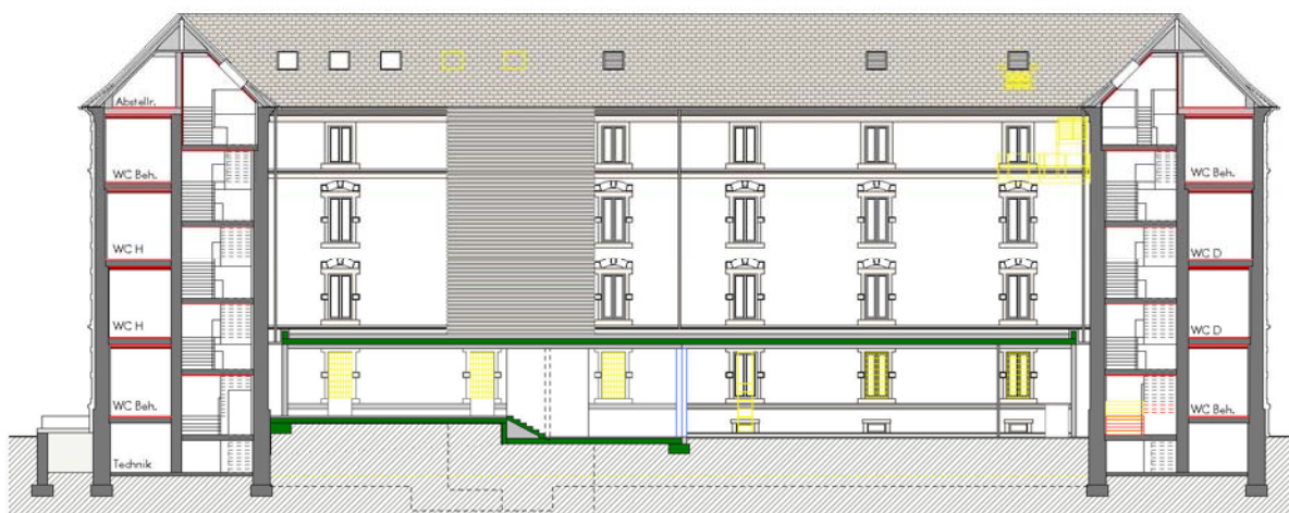
Schnitt E-E
