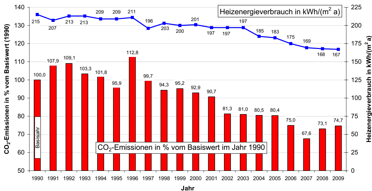
Abb. 1.3.2: Entwicklung des witterungsbereinigten Heizenergieverbrauchs und der CO 2 -Emissionen aller überwachten Liegenschaften der Stadt Karlsruhe von 1990 bis 2009 (normiert auf die Nettogrundfläche, Basis 1990 entspricht 100%).
