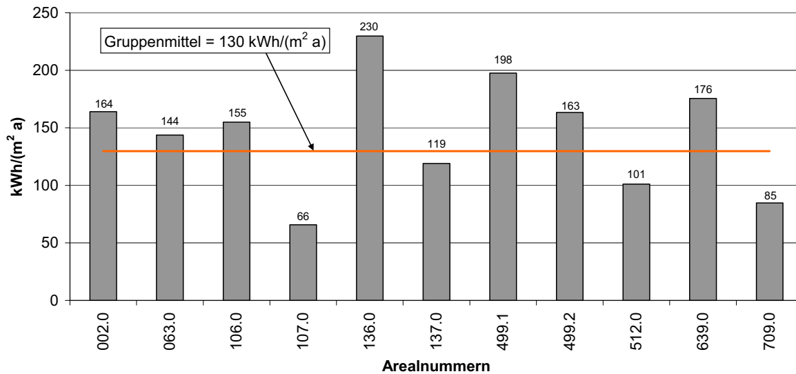
Heizenergiekennzahlen 2009 Hauswirtschaftliche, Kaufmännische und Gewerbliche Schulen (G)
