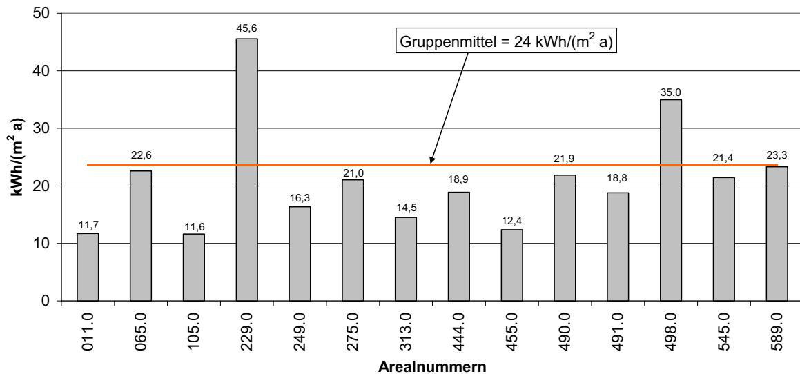
Stromkennzahlen 2009 Gymnasien (F)
