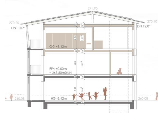
Schnitt A-A
