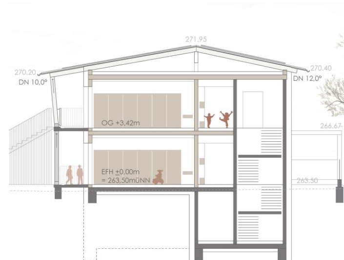
Schnitt B-B
