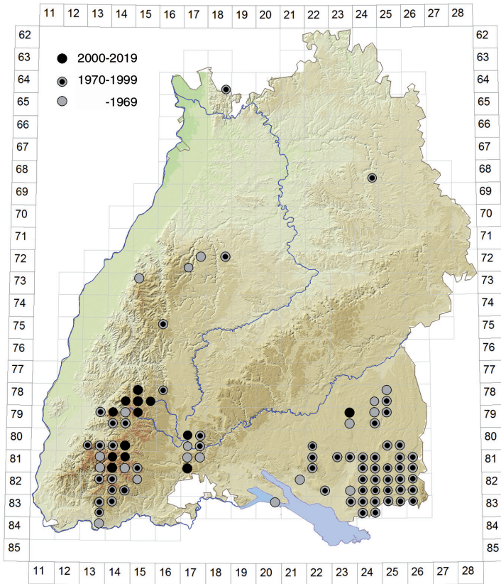
Abb. 9: Arealregression beim Moorigwiesenvögelchen Coenonympha tullia (Müller, 1764) in Baden-Württemberg. Mit der Jahrtausendwende ist die Art in Oberschwaben aus der Fläche fast verschwunden. – Quelle: Landesdatenbank Schmetterlinge Baden-Württembergs, Grafik aus InsectIS (© G. SEIGER). Fig. 9: Areal regression in the Large Heath Coenonympha tullia (Müller, 1764) in Baden-Württemberg. With the turn of the millennium the species had almost completely disappeared from the pre-alpine region Upper Swabia. – Source: central Lepidoptera database Baden-Wuerttemberg, graphic from InsectIS (© G. SEIGER).
