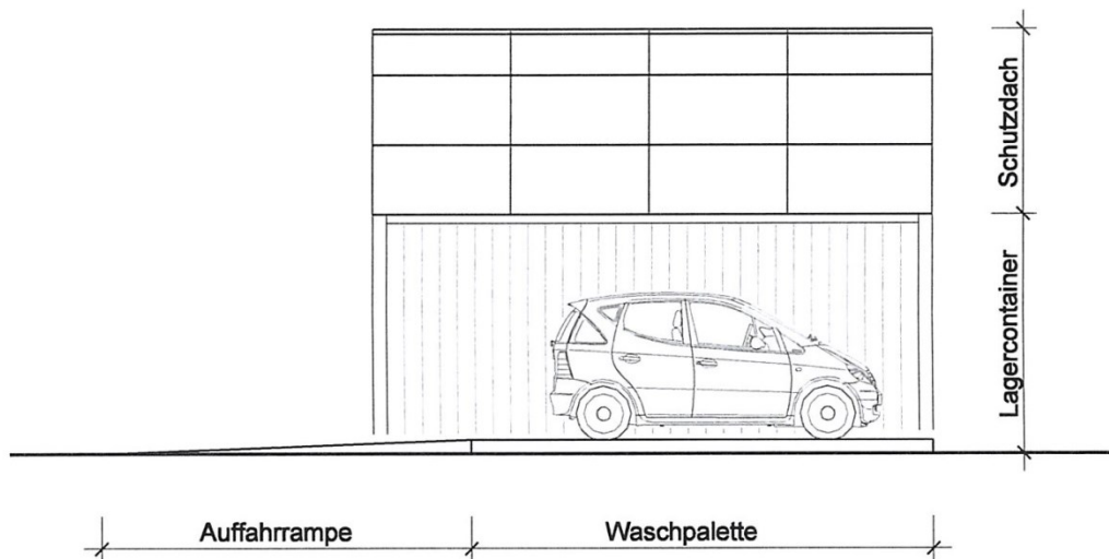
Schnitt A-A
