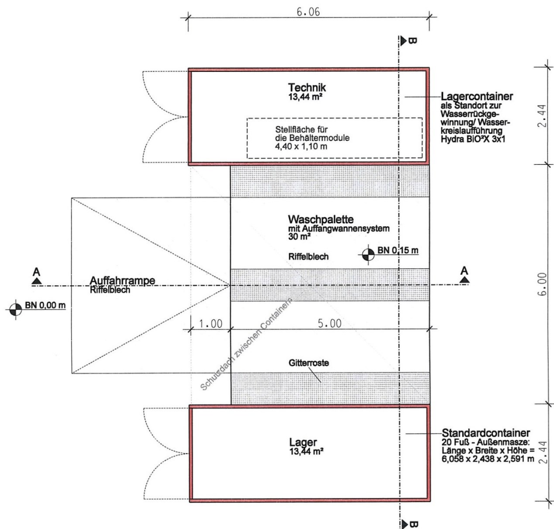
Grundriss Waschpalette
