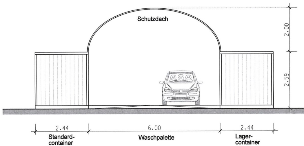
Ansicht Nord
