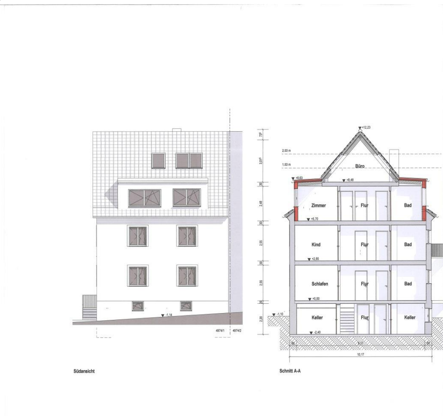
Ansicht Süd sowie Schnitt A-A
