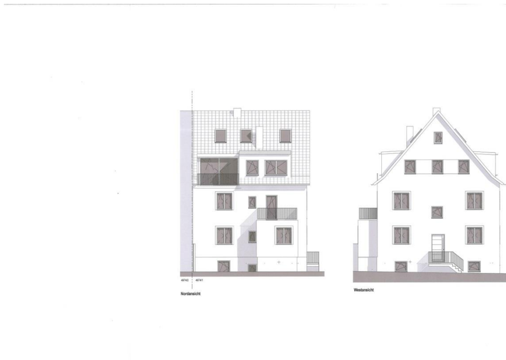
Ansicht Nord und West
