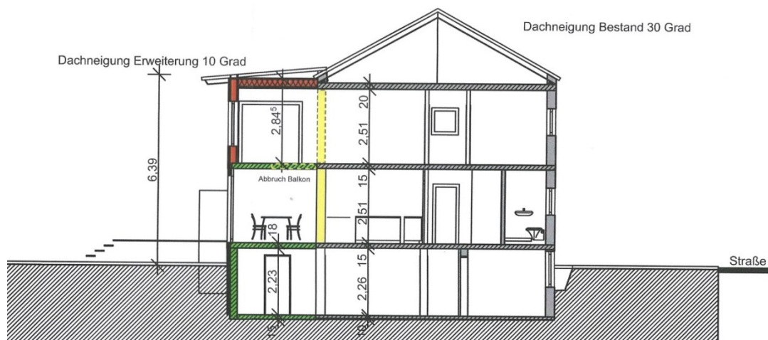
Schnitt
