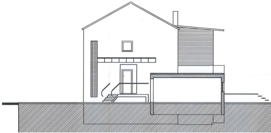
Ansicht Ost
