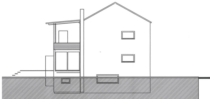
Ansicht West
