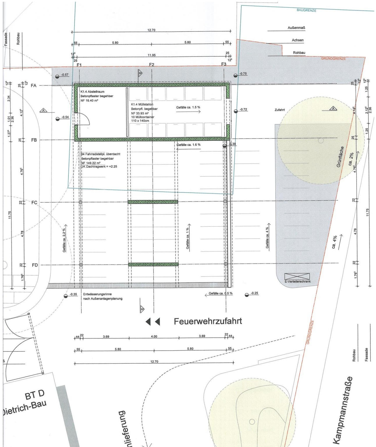
Grundriss
