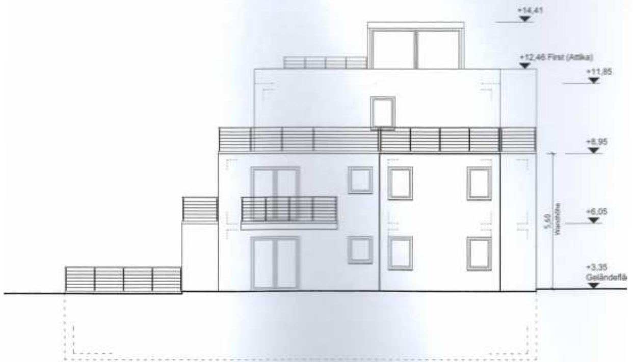
ANSICHT SÜD
