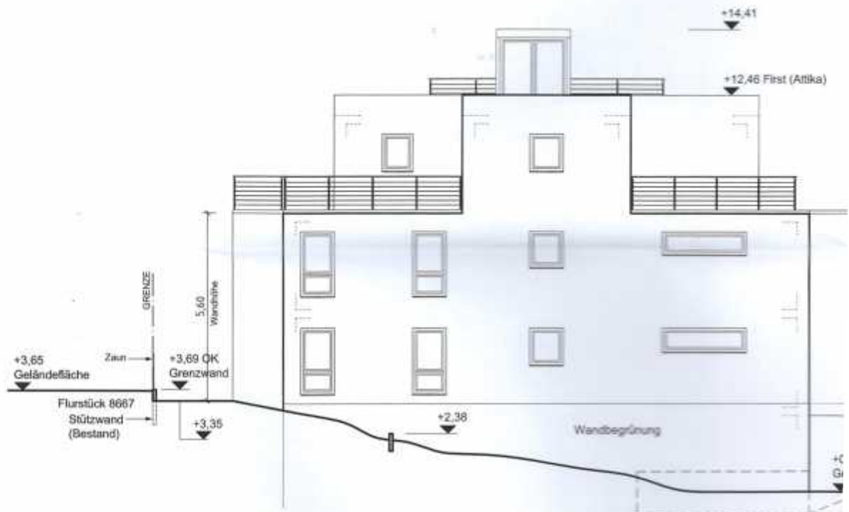
ANSICHT OST
