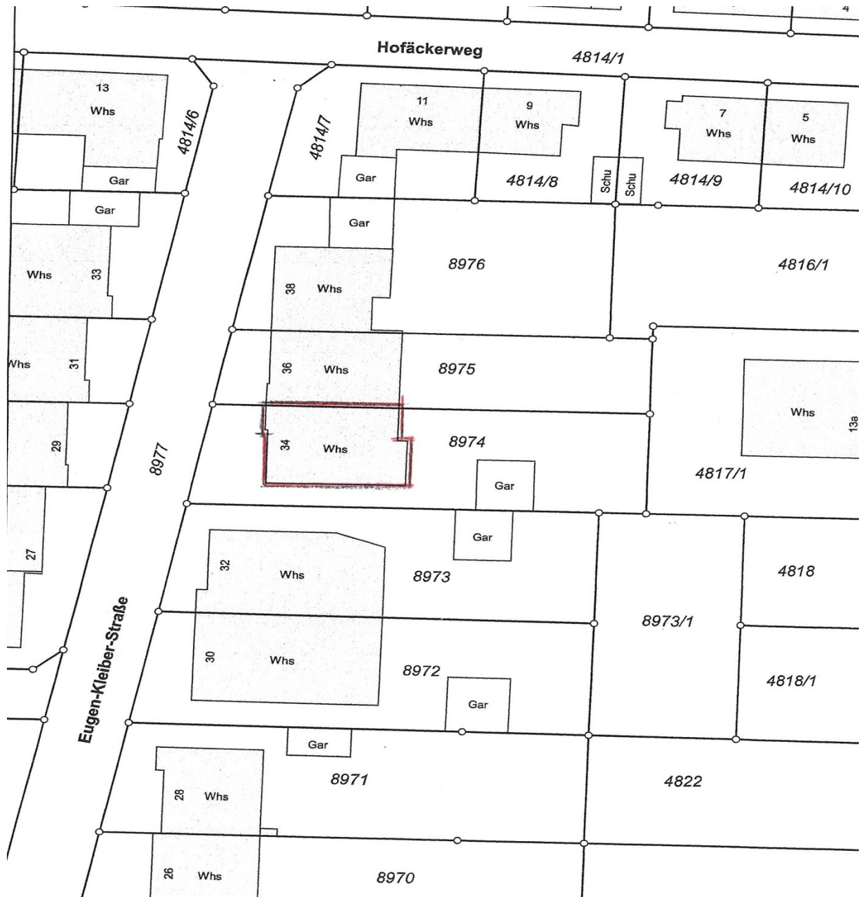
Lageplan
