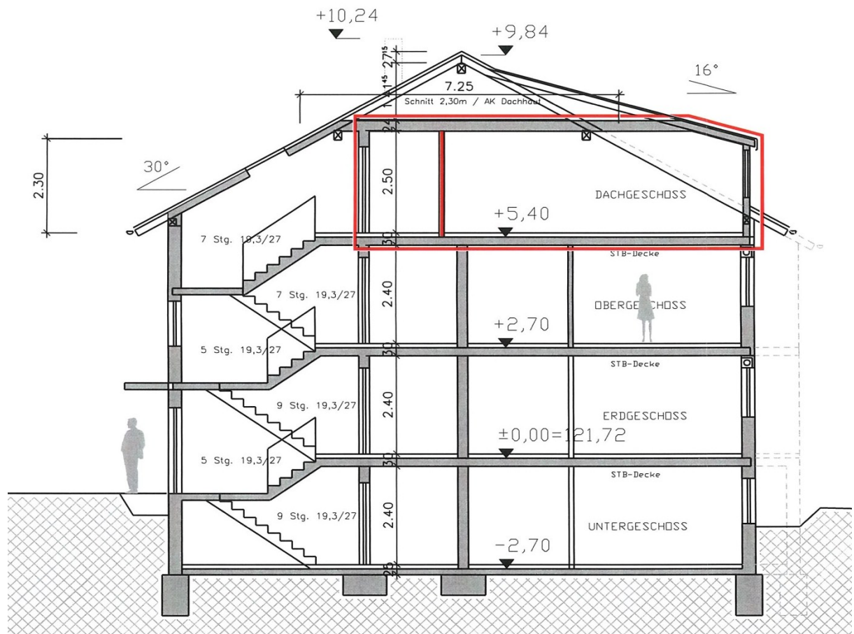
Schnitt
