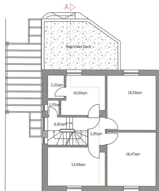
Grundriss 1.OG
