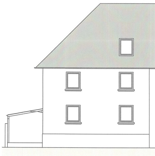
Ansicht Süd
