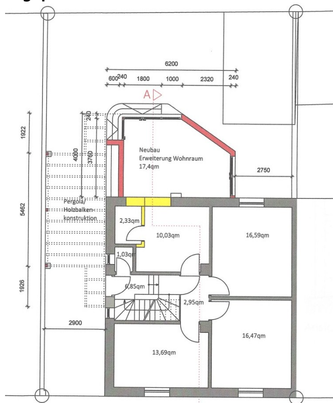
Grundriss EG
