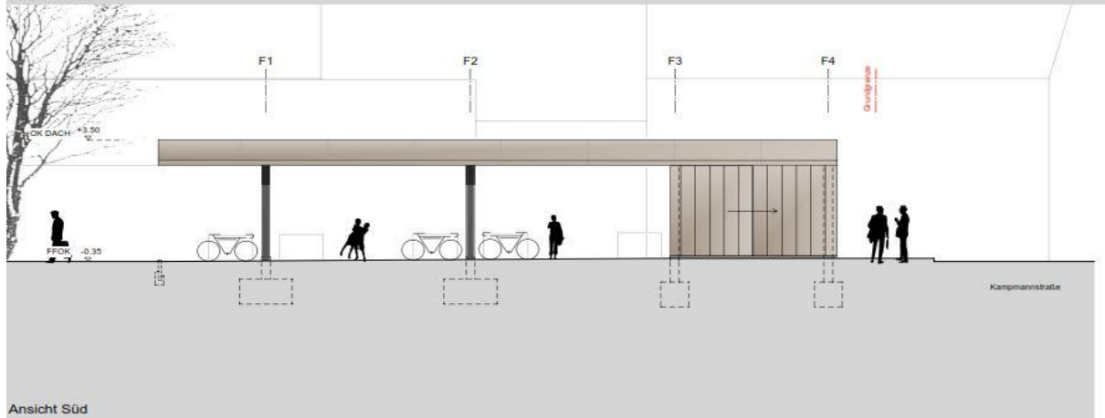
Ansicht Süd
