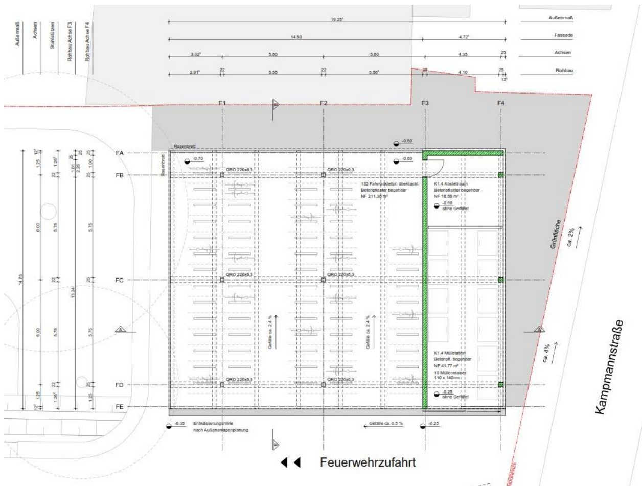
Grundriss überdachte Fahrradabstellplätze
