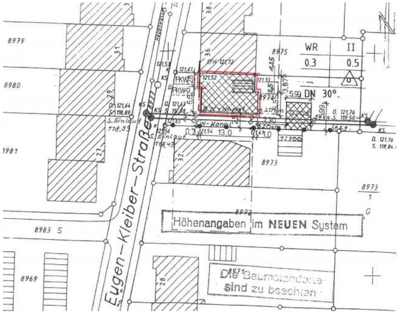
Lageplan
