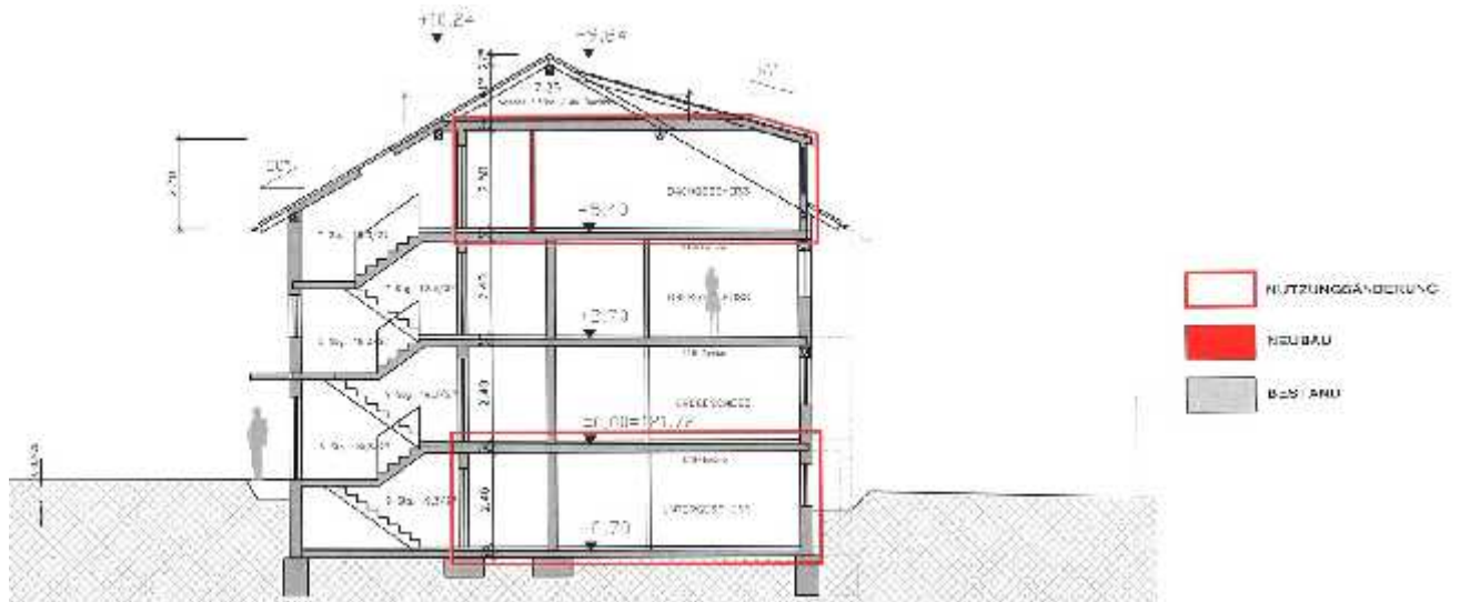
Schnitt
