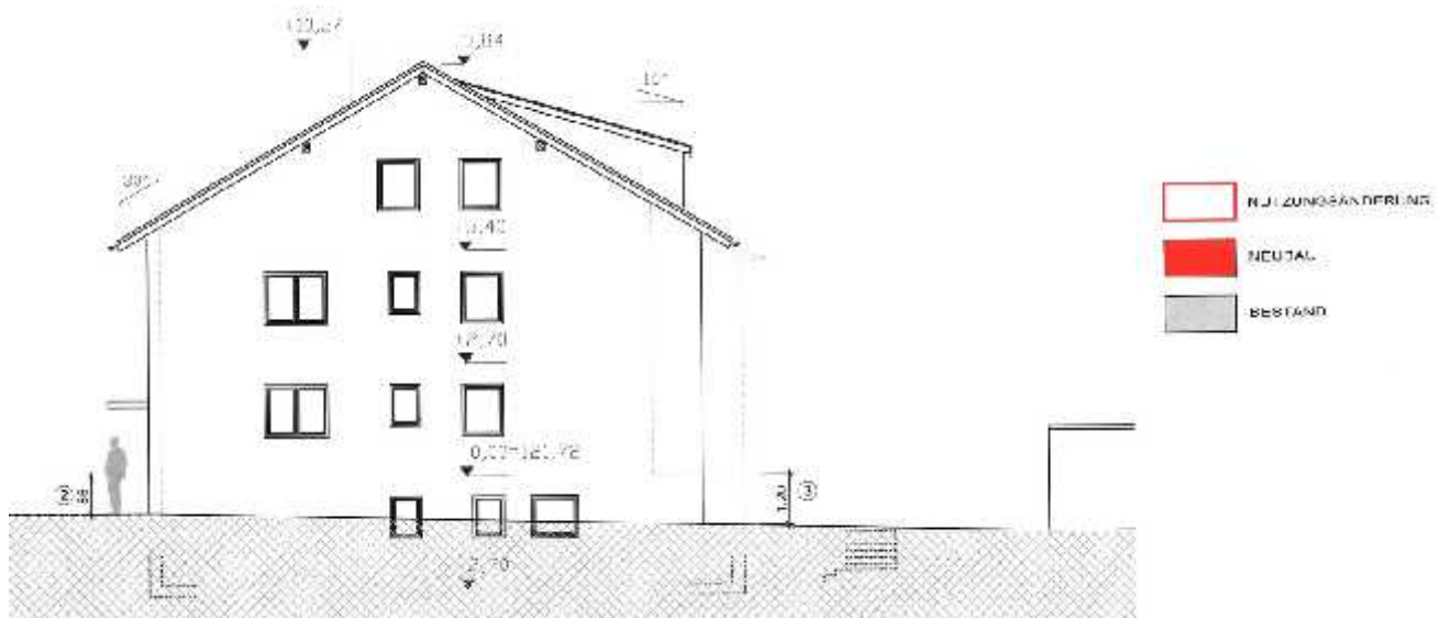
Ansicht Süd
