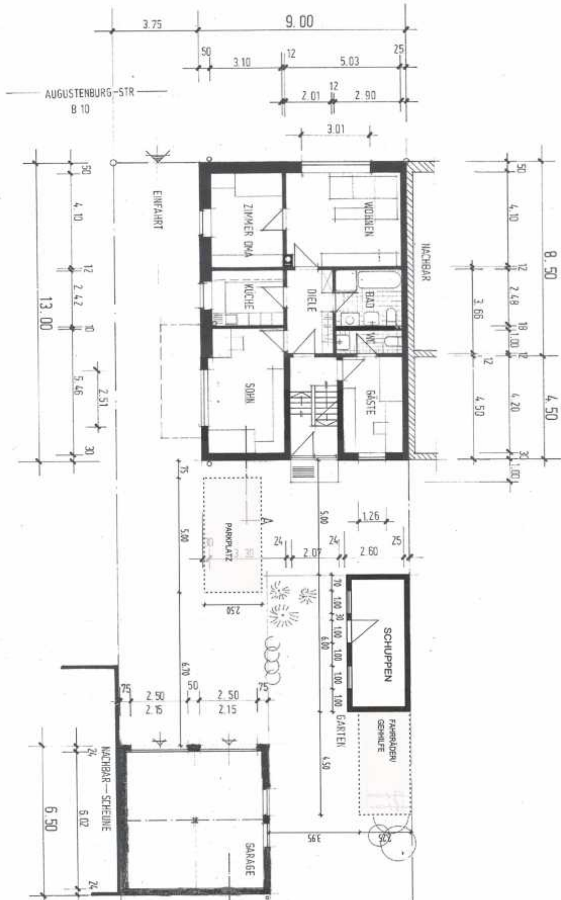
Grundriss EG
