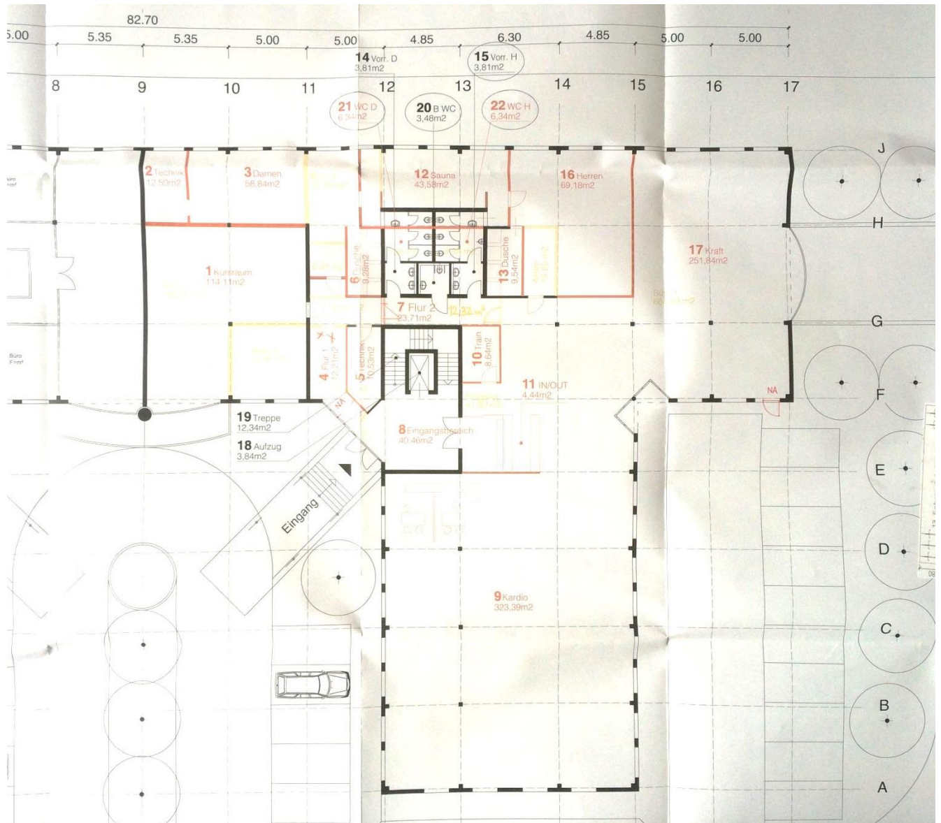
Grundriss EG Bauteil A
