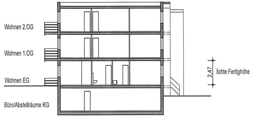
Schnitt 1-1
