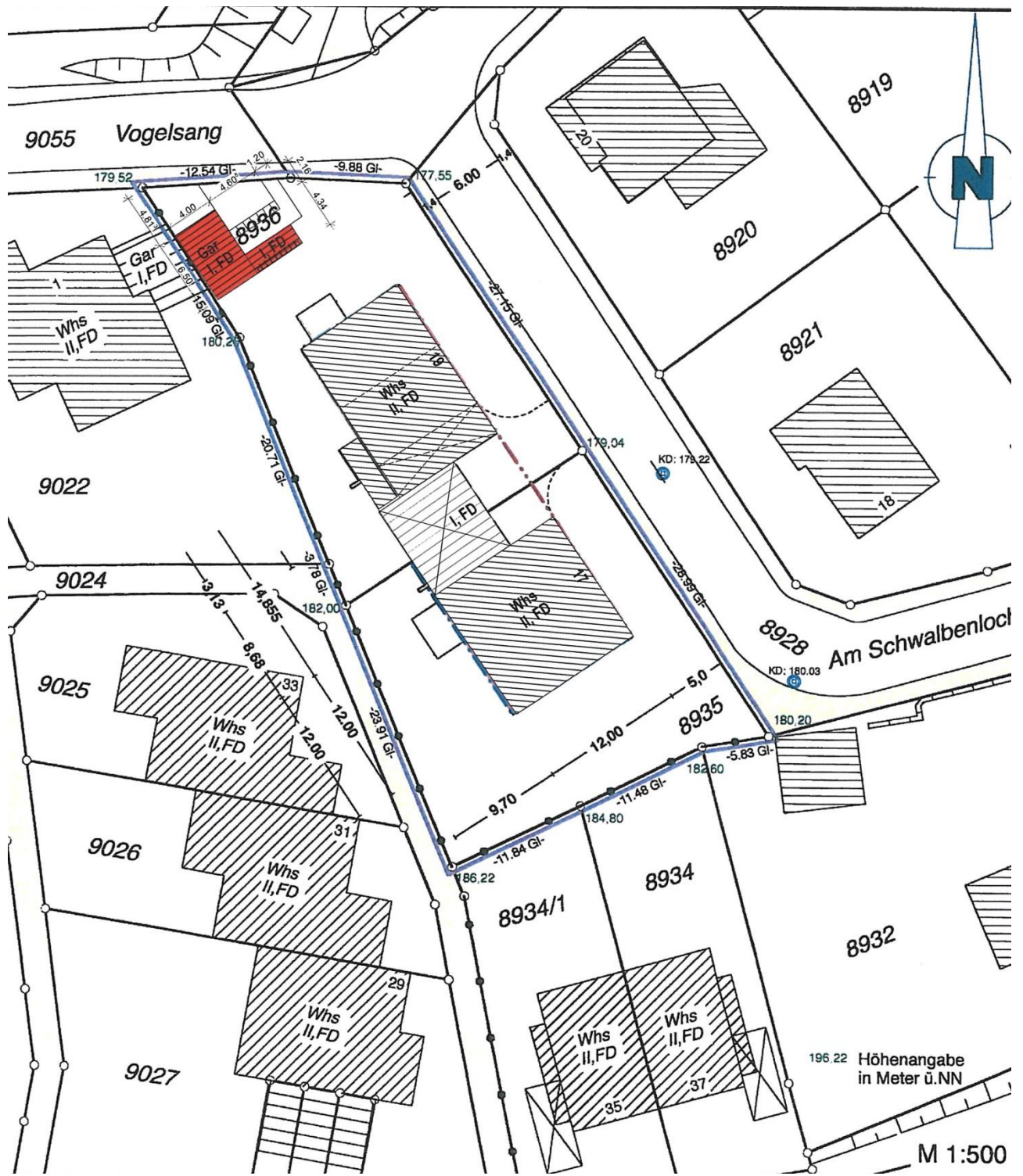
Lageplan
