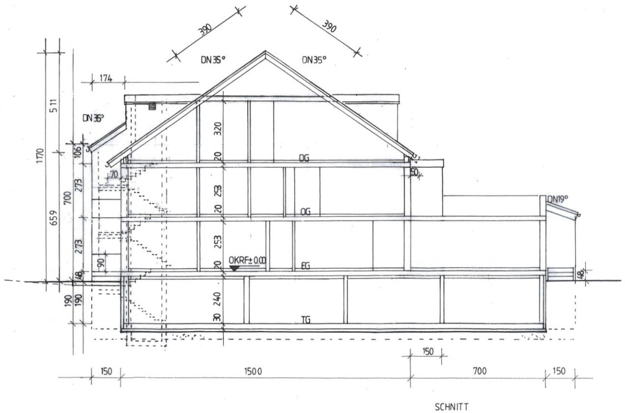
Schnitt
