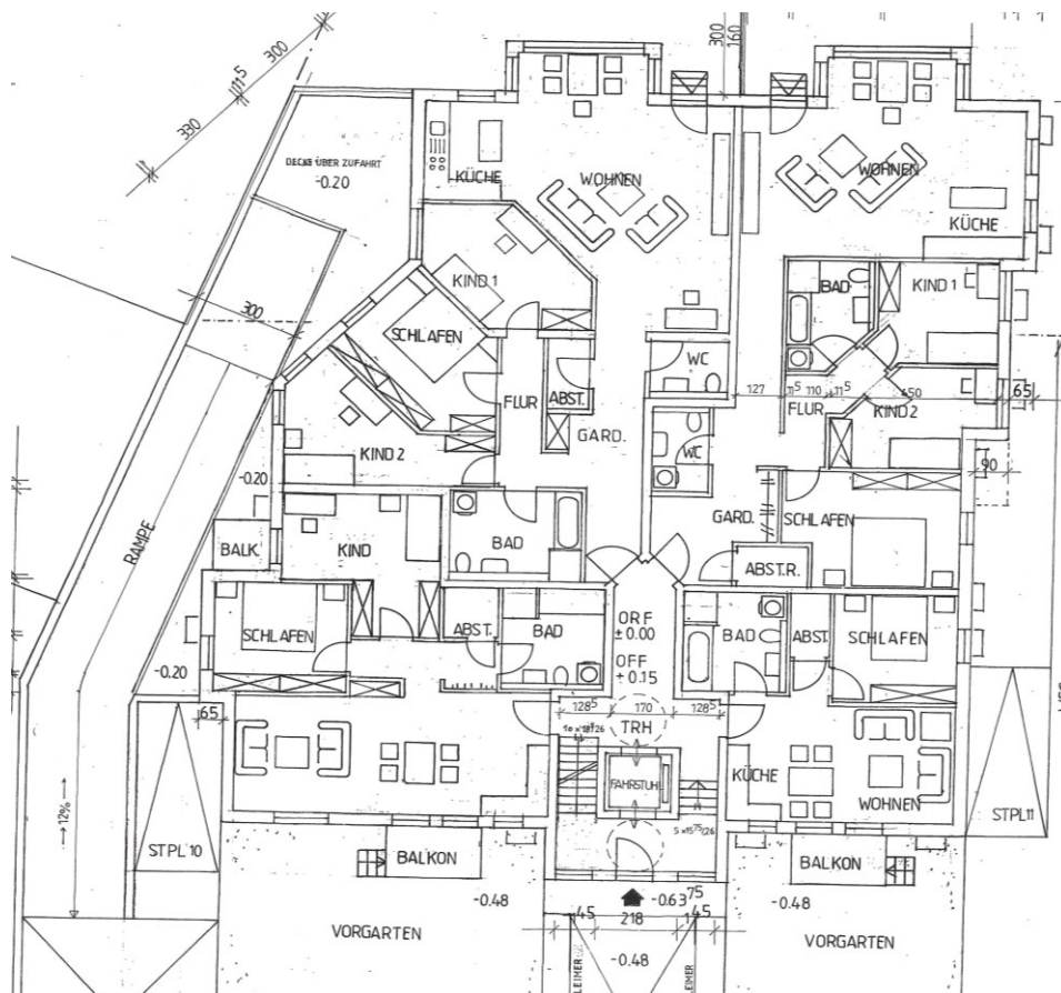
EG Grundriss
