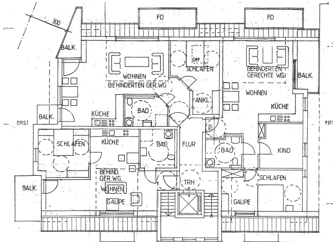
DG Grundriss
