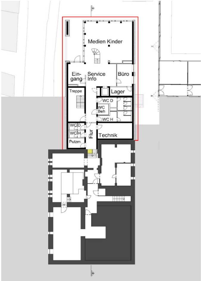
Bauteil A Untergeschoss
