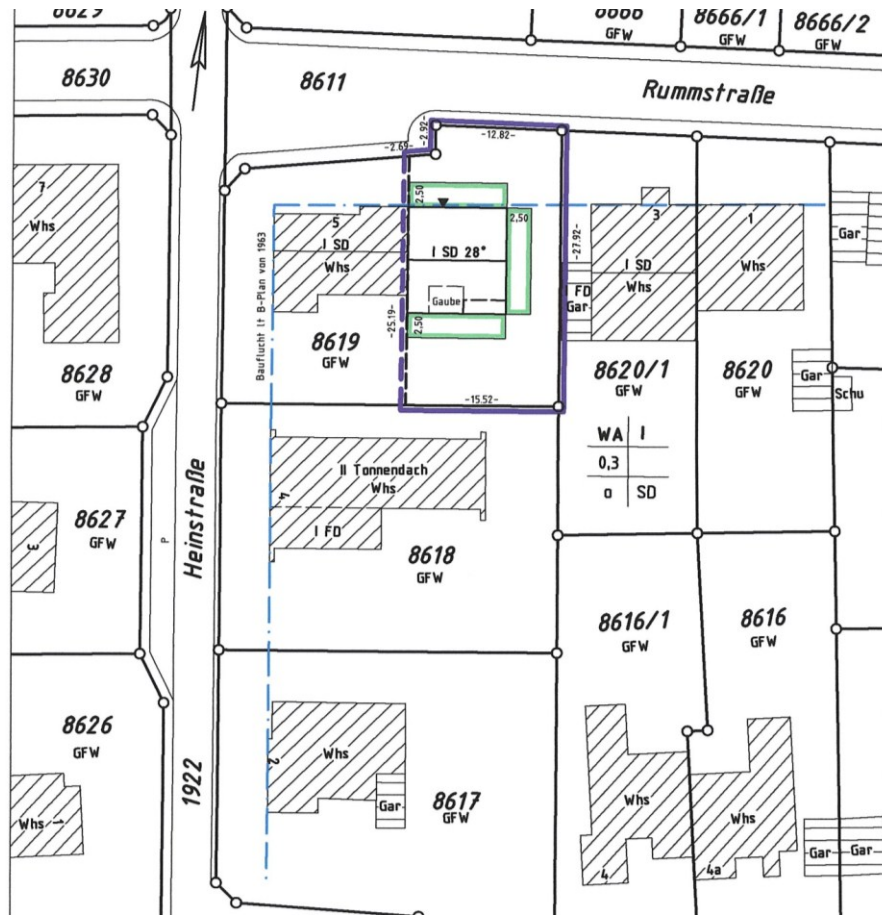
Abstandsflächenplan
