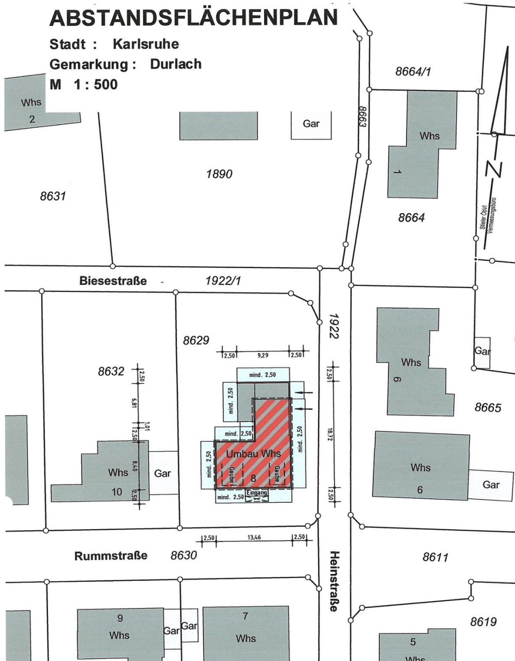
Abstandsflächenplan
