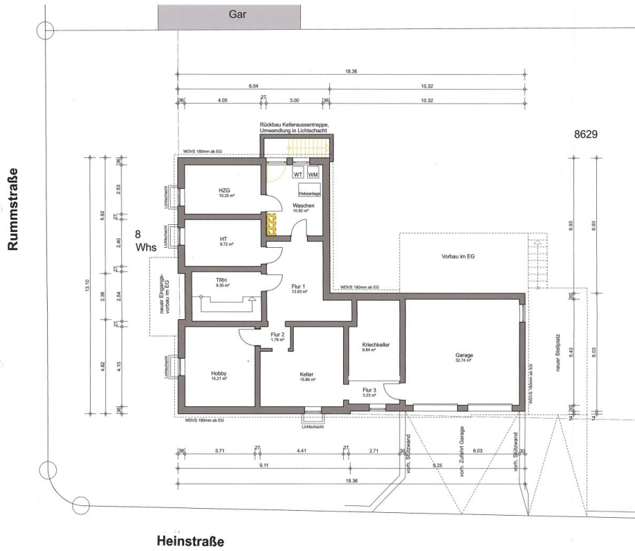
Grundriss UG
