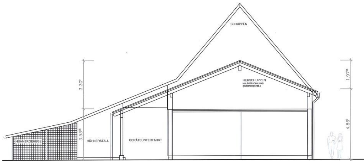
Ansicht Nord
