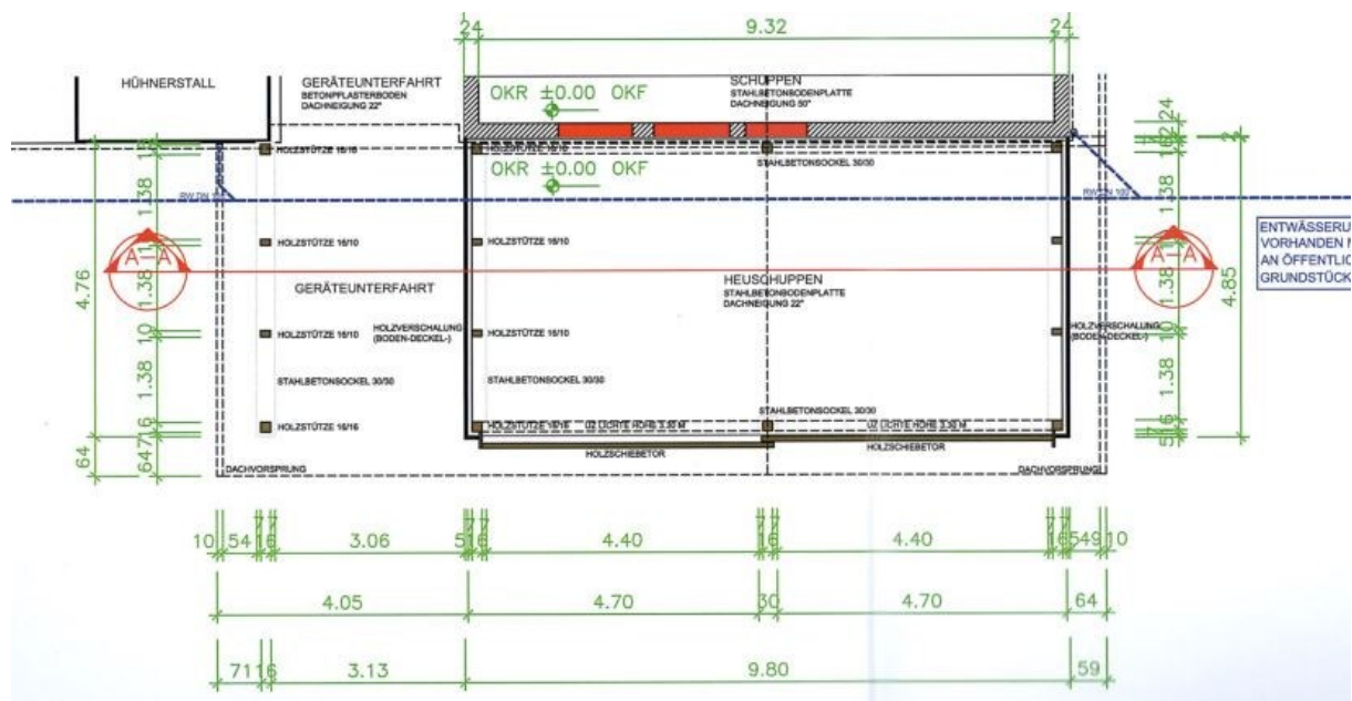
Grundriss
