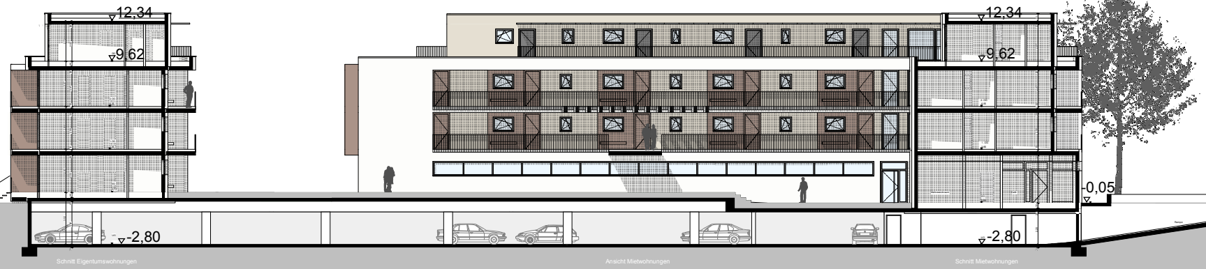
Schnitt 1, Innenansicht Südost
