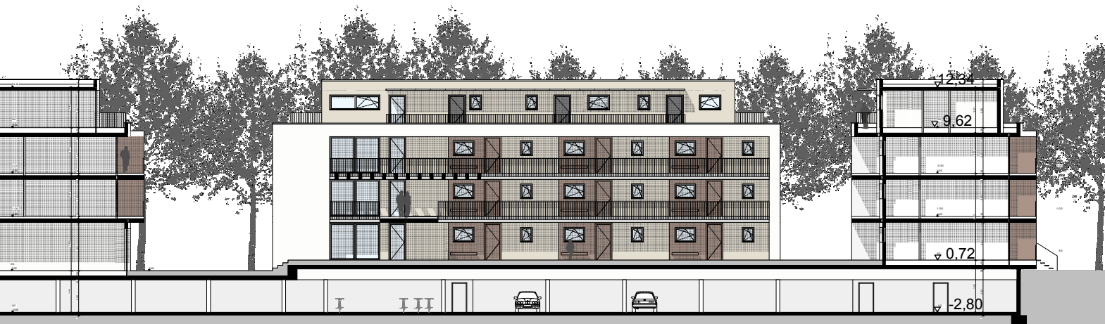
Schnitt 2, Innenansicht Nordwest Sophia
