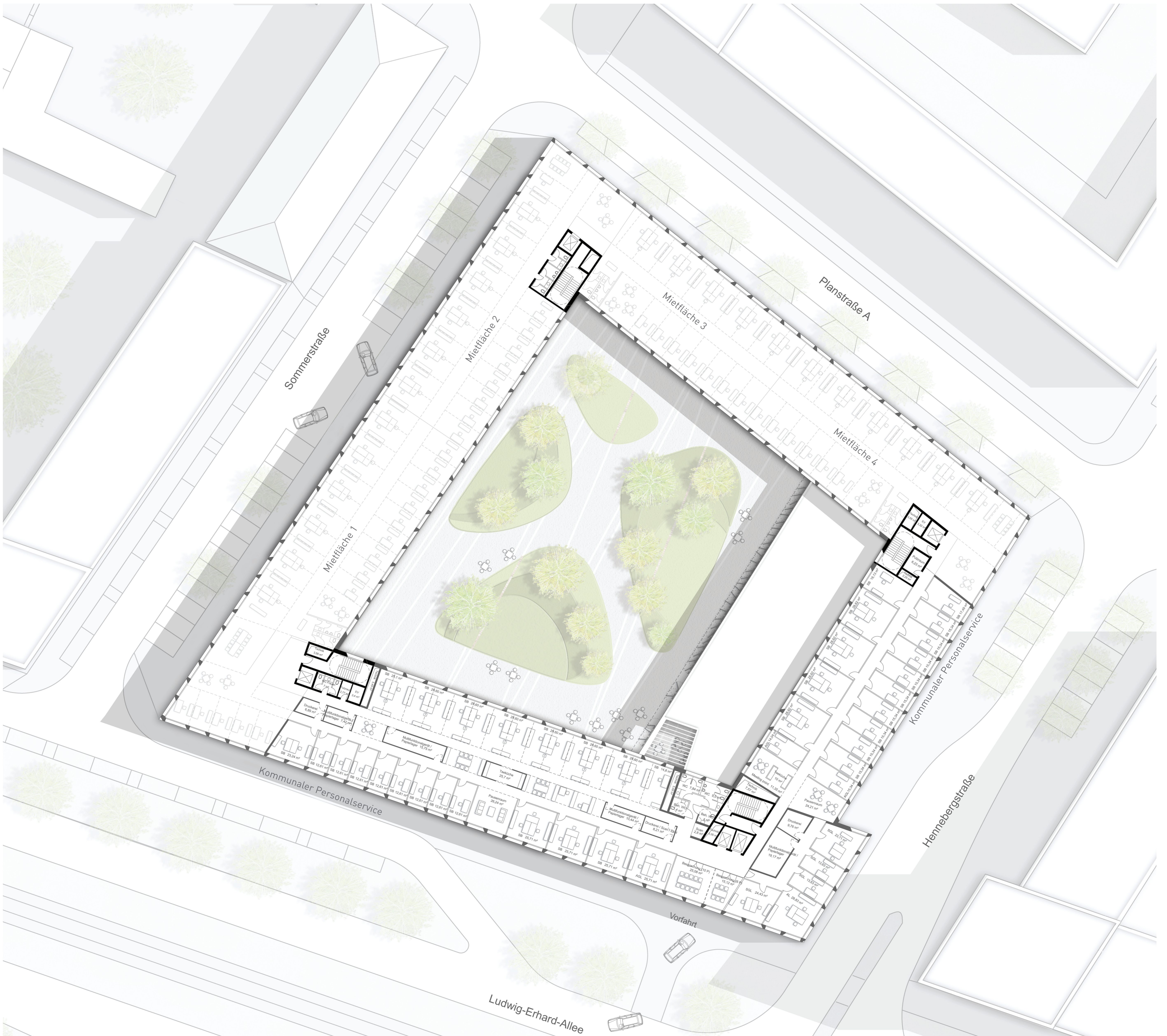
REGELGESCHOSS (2.OG) M. 1:200
